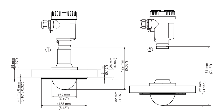
Fig. 90: NCR-86, sistema de antena blindado DN 80 PN 40
