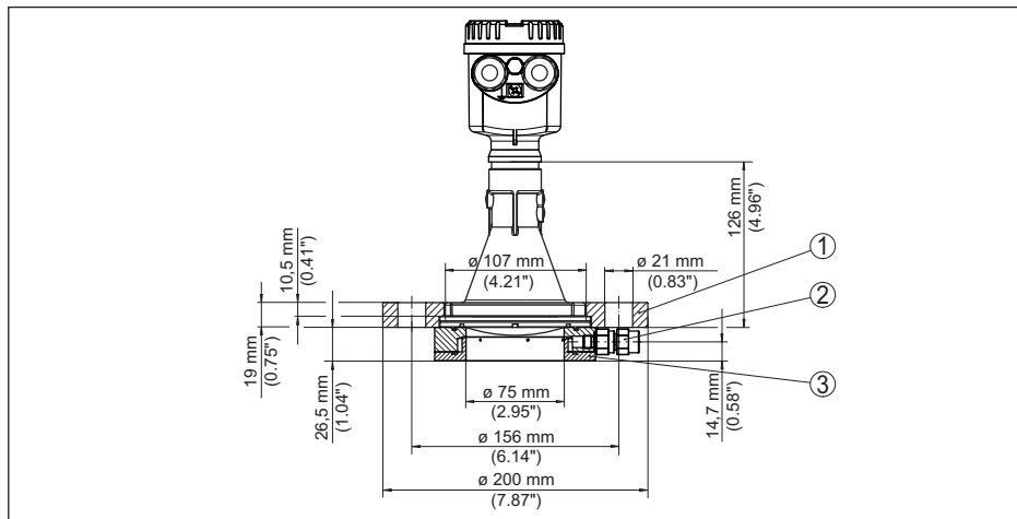
Fig. 79: NCR-86 com flange de capa e conexão de ar de limpeza adequado para 3" 150 lbs, DN 80 PN 16
