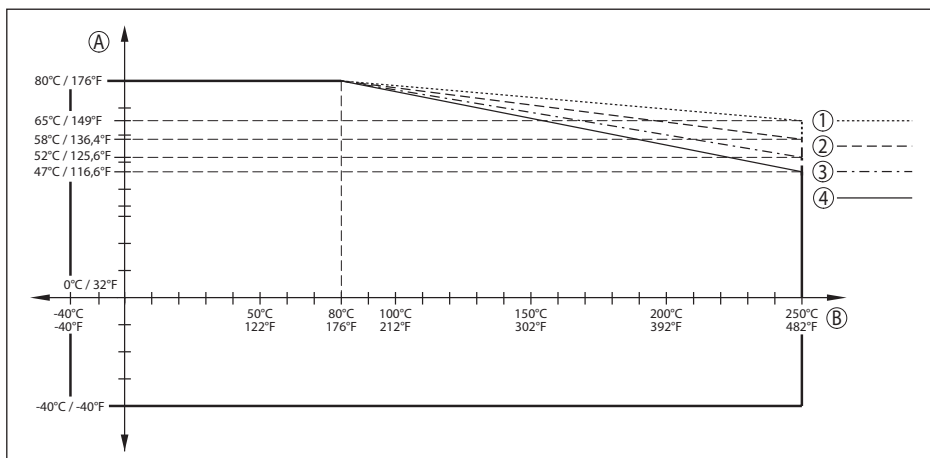
Fig. 70: Redução da temperatura ambiente, flange com antena lentiforme até +250 °C (+482 °F)
