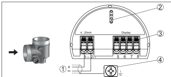
Fig. 47: Compartimento de conexão - Caixa de duas câmaras
