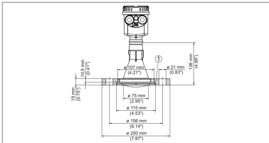
Fig. 78: NCR-86 com flange de capa adequado para 3" 150 lbs, DN 80 PN 16
