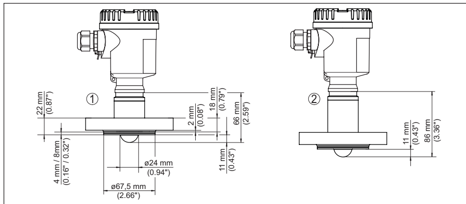
Fig. 89: NCR-86, sistema de antena blindado DN 25 PN 40
