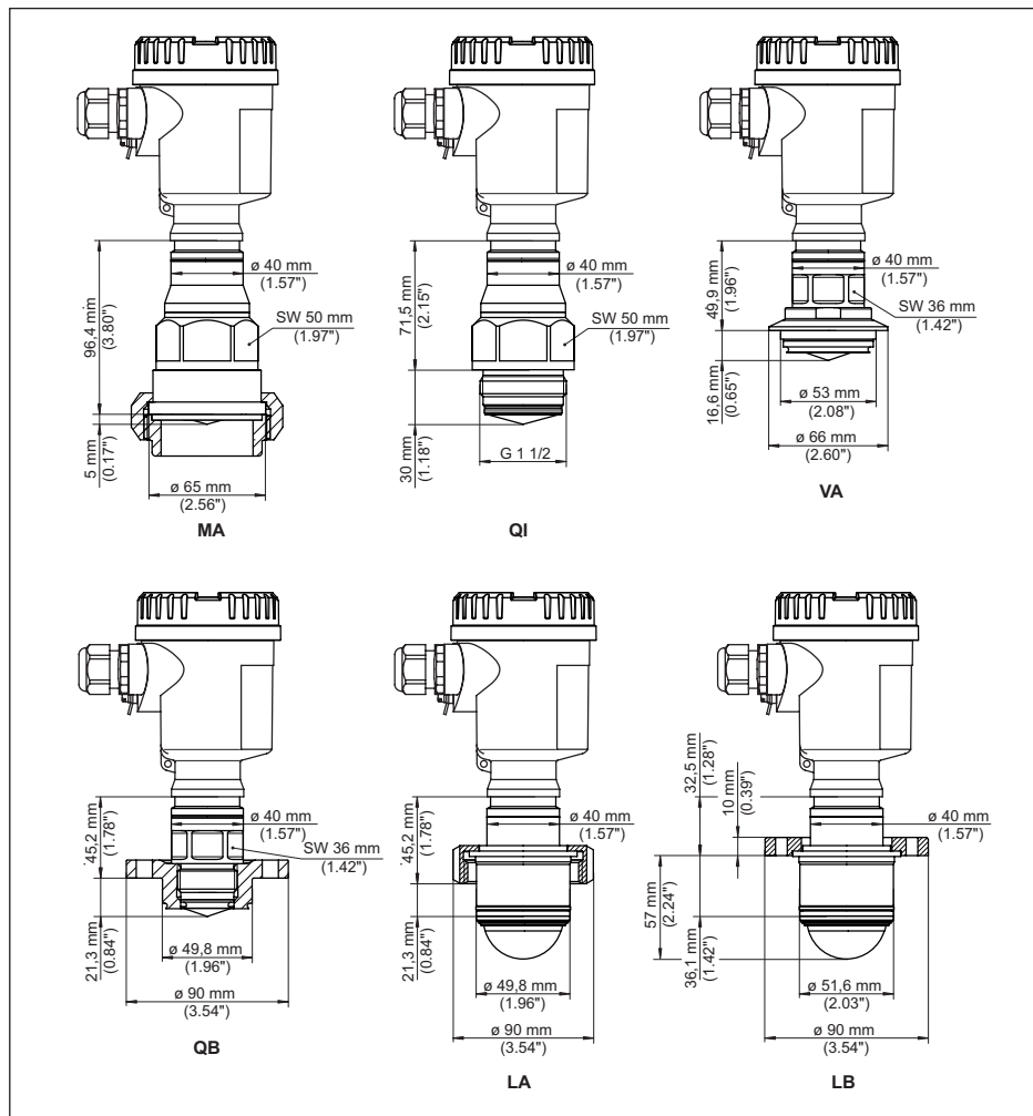
Fig. 93: NCR-86, conexão asséptica
