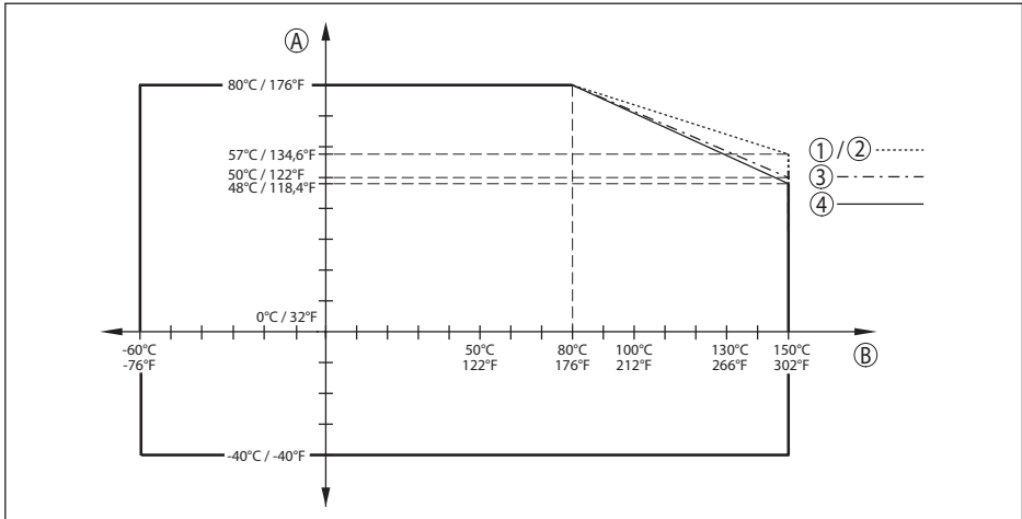
Fig. 65: Redução da temperatura ambiente, flange com sistema de antena encapsulado, -60 ... +150 °C (-76 ... +302 °F)
