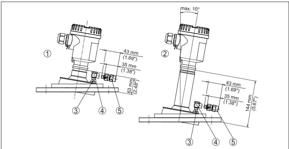
Fig. 97: NCR-86, flange com antena lentiforme, suporte giratório e conexão de ar de limpeza
