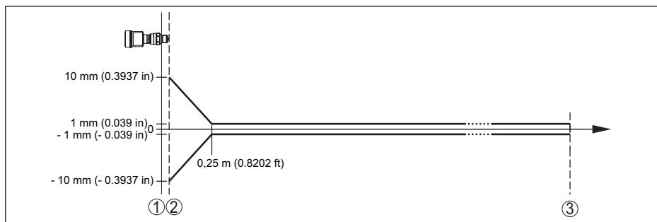
Fig. 59: Diferença de medição sob condições de referência (exemplo: rosca com sistema de antena integrado, vale da mesma forma para todos os modelos) 22)
