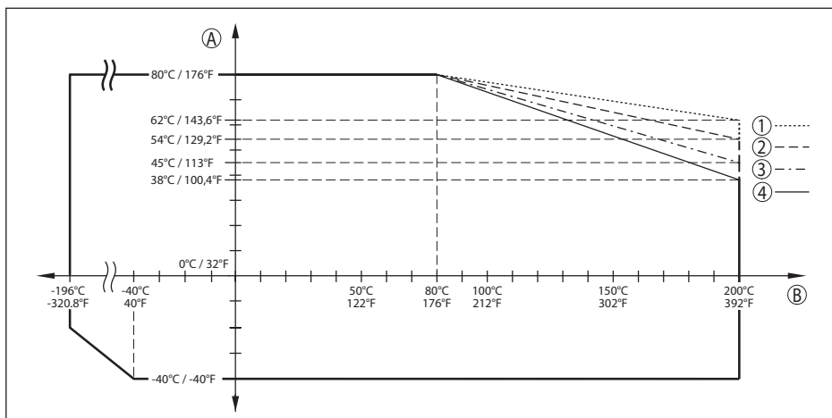
Fig. 67: Redução da temperatura ambiente, flange com sistema de antena encapsulado, -196 ... +200 °C (-320.8 ... +392 °F)
