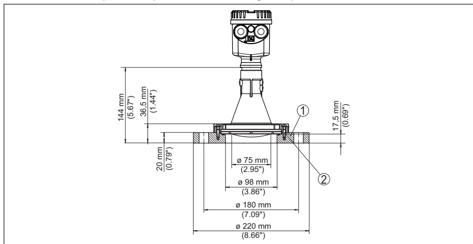
Fig. 80: NCR-86 com flange adaptador DN 100 PN 6
