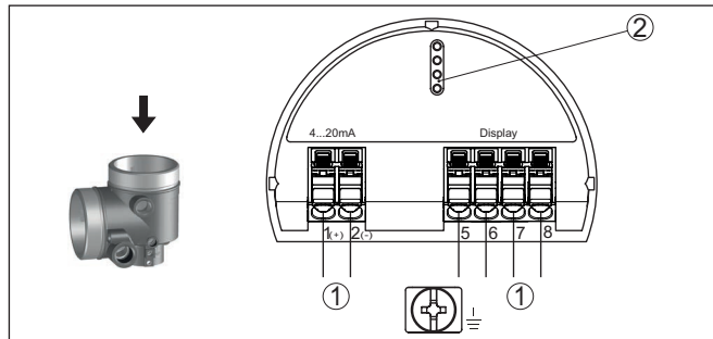
Fig. 46: Compartimento do sistema eletrônico - Caixa de duas câmaras
