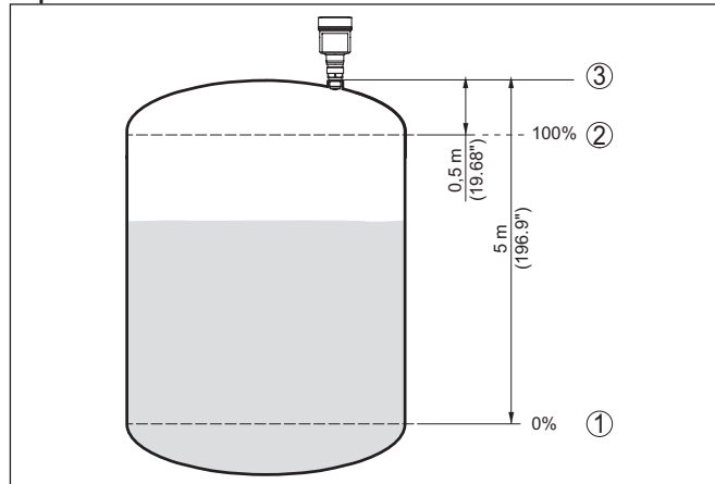
Fig. 52: Exemplo de parametrização calibração de Mín./Máx. - líquidos
