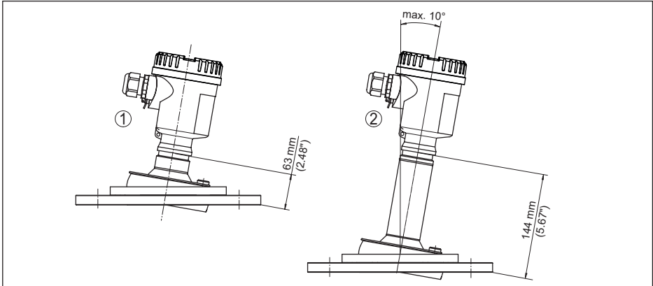
Fig. 96: NCR-86, flange com antena lentiforme e suporte giratório
