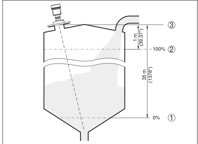
Fig. 53: Exemplo de parametrização calibração de Min./Máx. - sólidos
