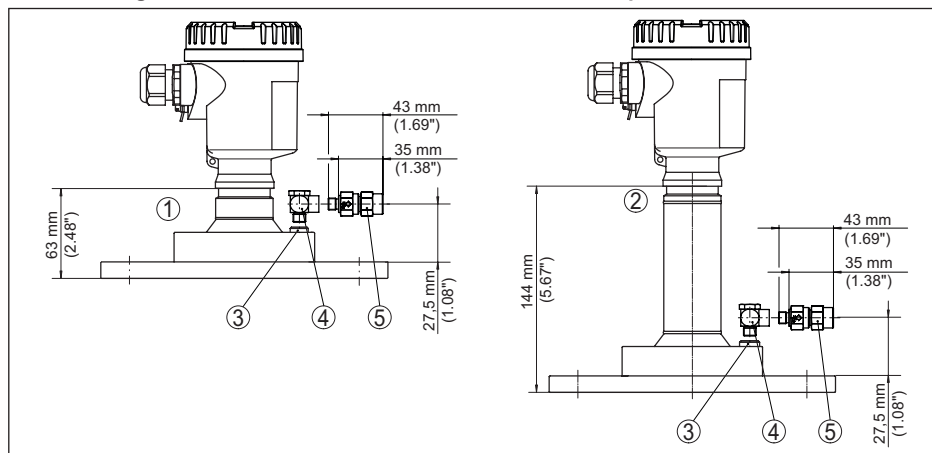
Fig. 95: NCR-86, flange com antena lentiforme e conexão de ar de limpeza
