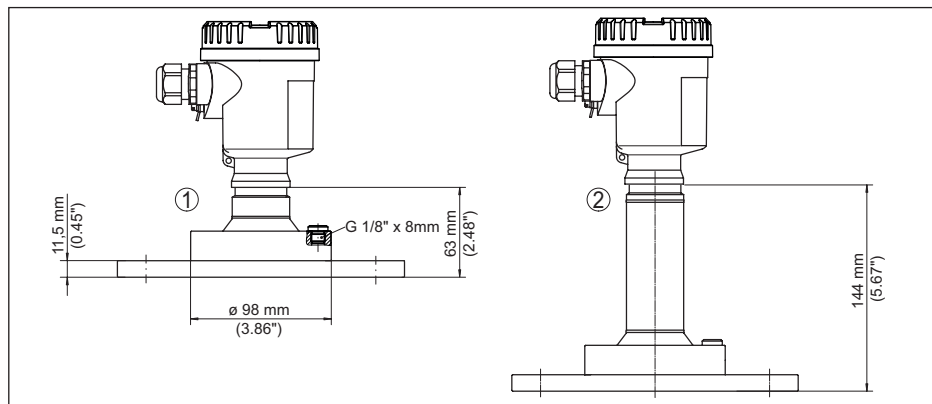
Fig. 94: NCR-86, flange com antena lentiforme (espessura do flange, vide desenho, tamanho do flange conforme DIN, ASME, JIS)
