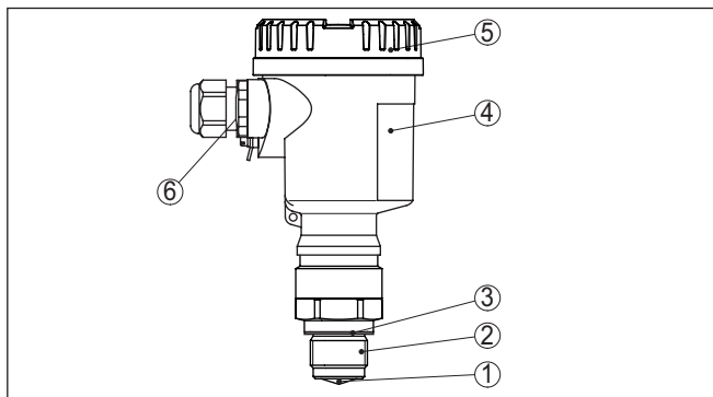
Fig. 1: Componentes do NCR-86
