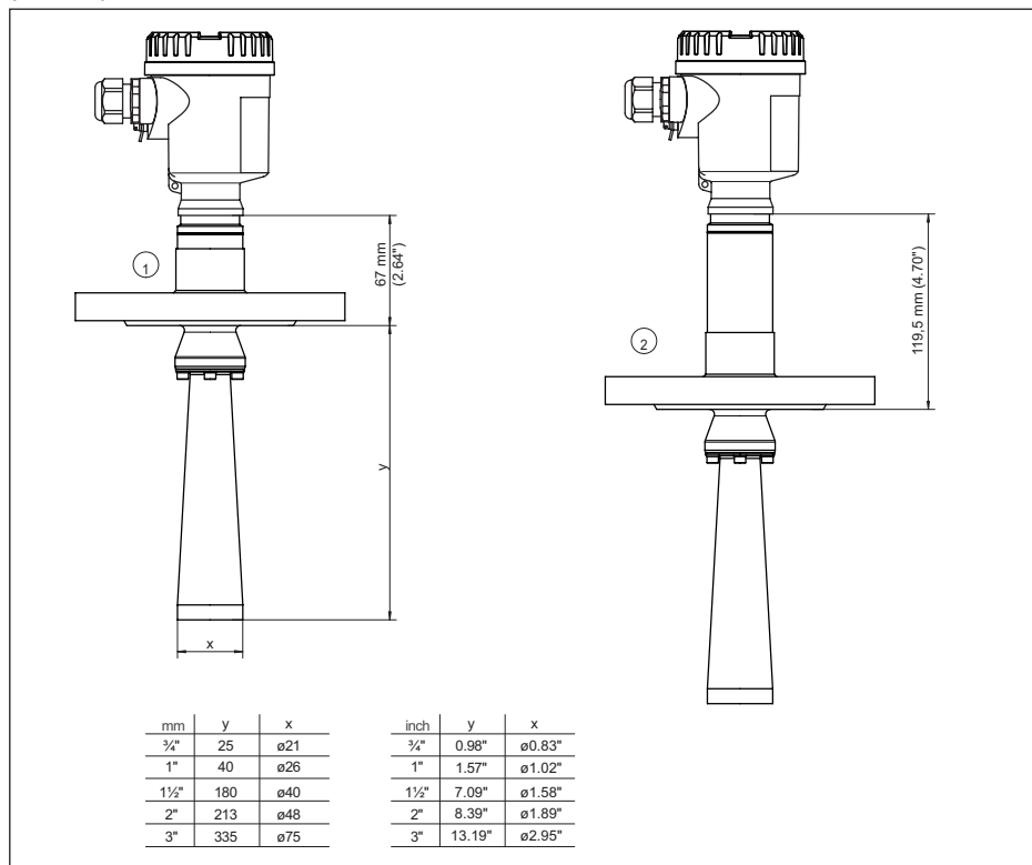
Fig. 86: NCR-86, flange com antena tipo corneta até +150 °C (+302 °F)/+250 °C (+482 °F)
