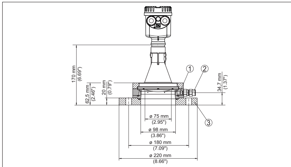
Fig. 81: NCR-86, flange adaptador e conexão de ar de limpeza DN 100 PN 6
