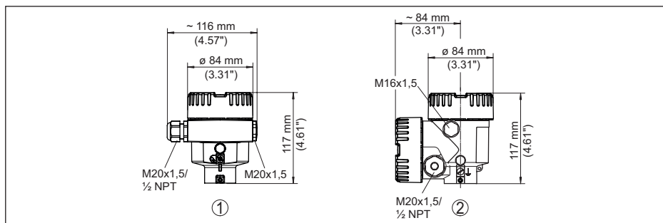
Fig. 76: Variantes da caixa com grau de proteção IP66/IP68 (0,2 bar), (com o módulo de visualização e configuração montado, a altura da caixa é aumentada em 18 mm/0.71 in)
