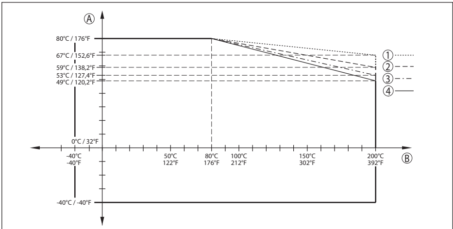
Fig. 73: Redução da temperatura ambiente, flange com antena tipo corneta até +200 °C (+392 °F)
