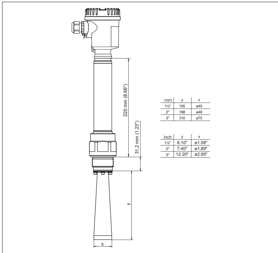
Fig. 87: NCR-86, rosca com antena tipo corneta modelo 450 °C
