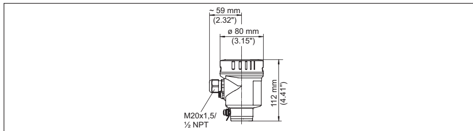
Fig. 77: Variantes da caixa com grau de proteção IP66/IP68 (0,2 bar), (com o módulo de visualização e configuração montado, a altura da caixa é aumentada em 18 mm/0.71 in)
