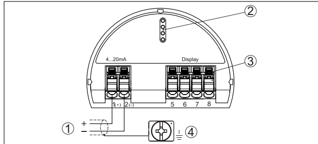
Fig. 45: Compartimento do sistema eletrônico e de conexões - Caixa de uma câmara
