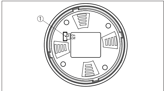
Fig. 54: Ativar Bluetooth
