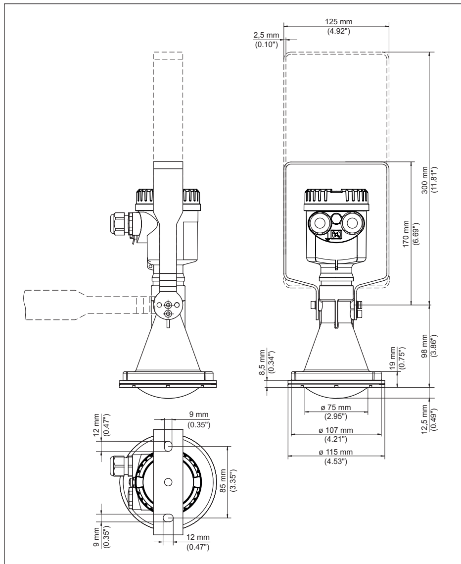
Fig. 82: NCR-86, antena de plástico tipo corneta, suporte de montagem com 170 ou 300 mm de comprimento
