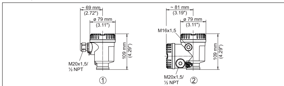
Fig. 75: Variantes da caixa com proteção IP66/IP67 (com o módulo de leitura e comando montado, a altura da caixa é aumentada em 9 mm/0,35 in)
