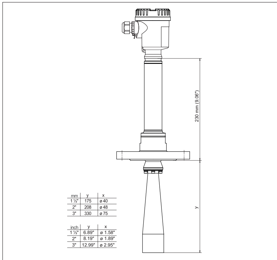
Fig. 88: NCR-86, flange com antena tipo corneta modelo 450 °C
