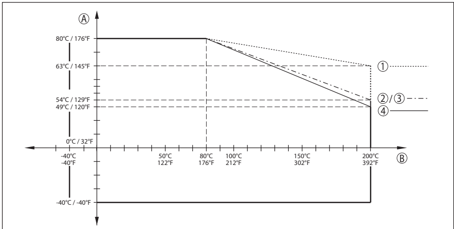
Fig. 69: Redução da temperatura ambiente, flange com antena lentiforme até +200 °C (+392 °F)
