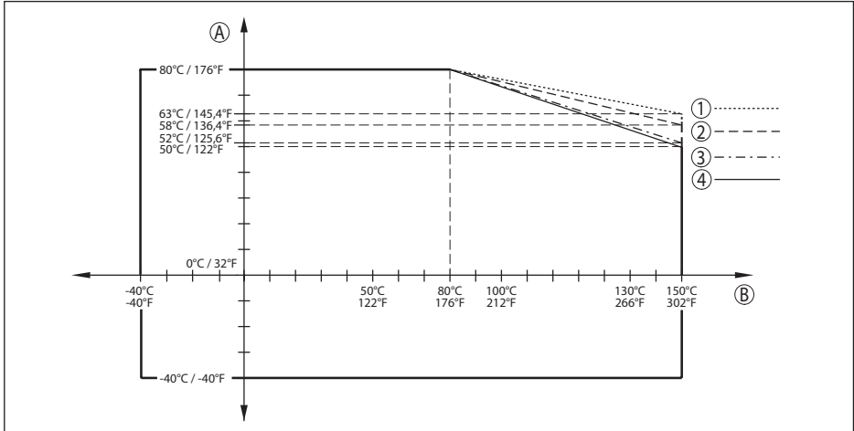
Fig. 68: Redução da temperatura ambiente, flange com antena lentiforme até +150 °C (+302 °F)
