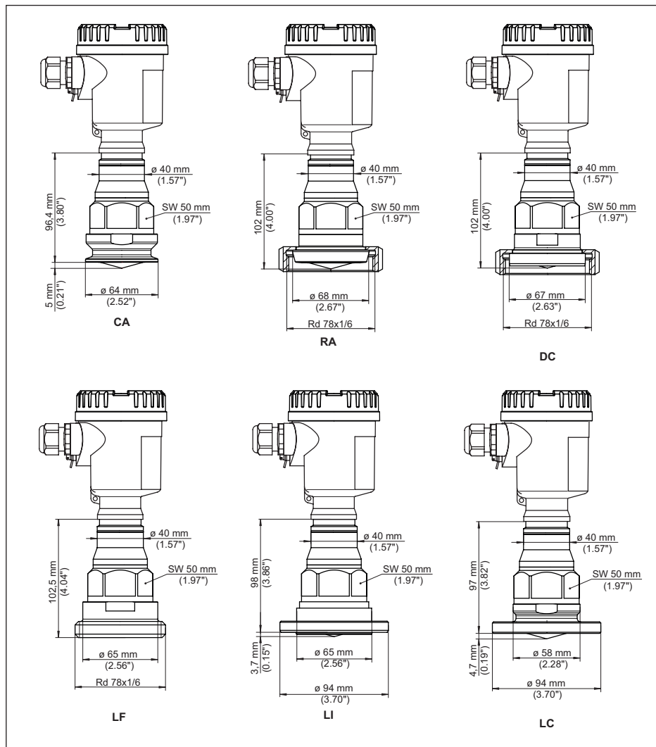
Fig. 92: NCR-86, conexão asséptica
