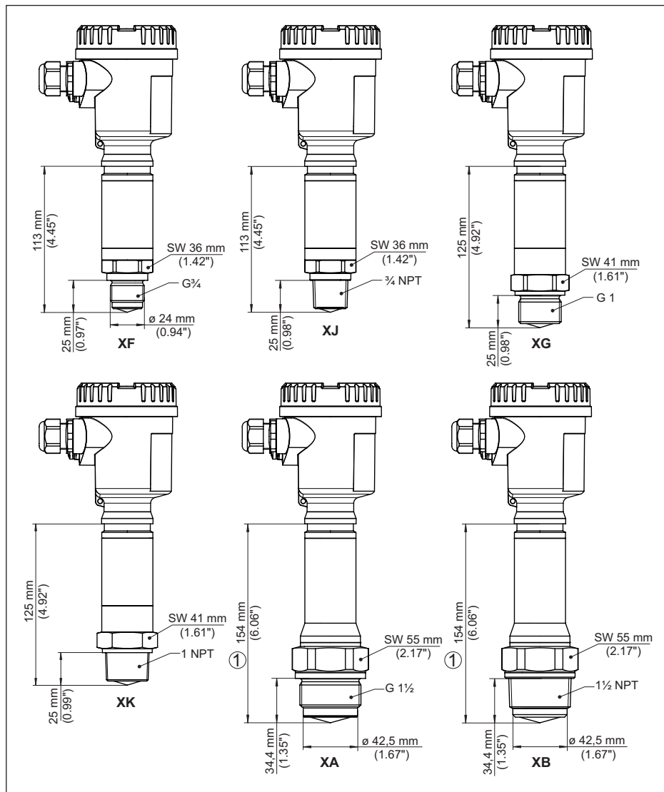
Fig. 85: NCR-86, rosca com sistema de antena integrado até +200 °C (+392 °F)/+250 °C (+482 °F)
