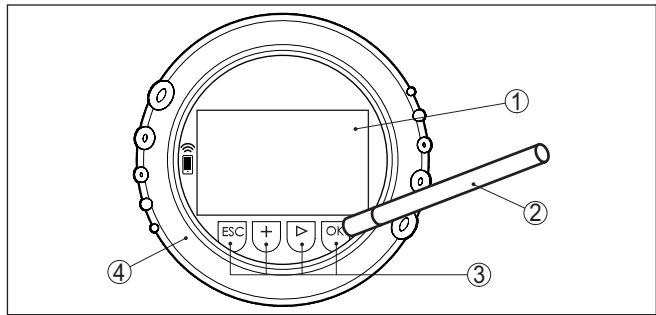
Fig. 51: elementos de visualização e configuração - com configuração por meio de caneta magnética
