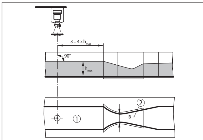
Fig. 43: Medição de débito com calha Venturi Kha-fagi : h_{m\acute{a}x.} = enchimento máx. da calha; B = maior estrangulamento da calha
