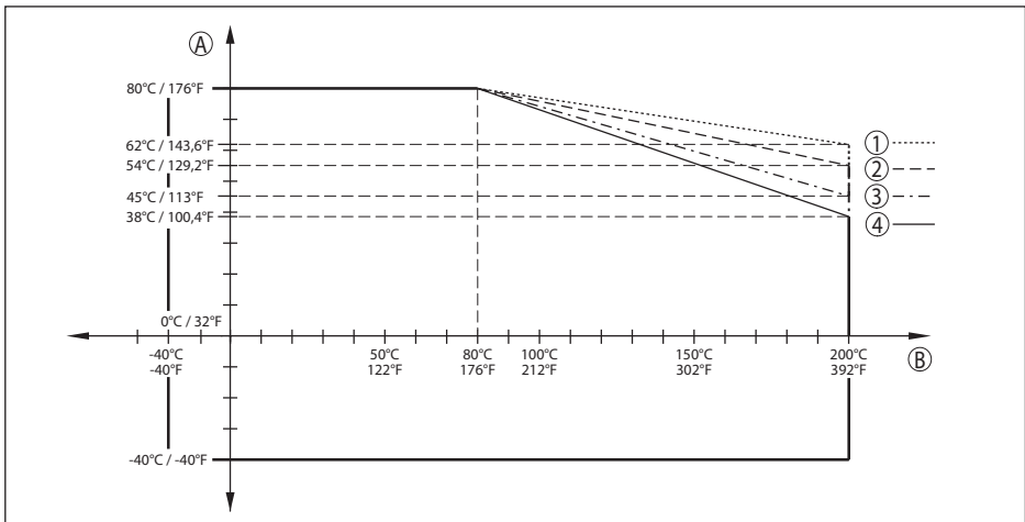
Fig. 66: Redução da temperatura ambiente, flange com sistema de antena encapsulado até +200 °C (+392 °F)
