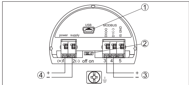
Abb. 7: Anschlussraum
