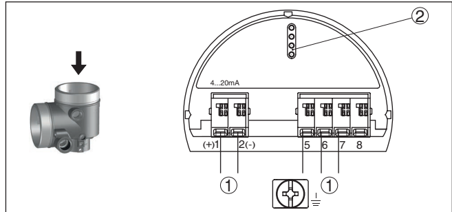
Fig. 6: Compartiment électronique - boîtier à deux chambres
