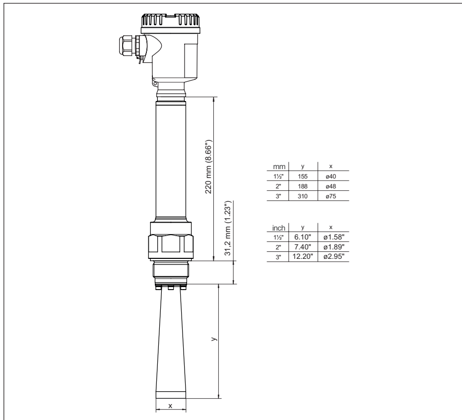
Fig. 87: NCR-86, rosca con antena de trompeta versión 450 °C
