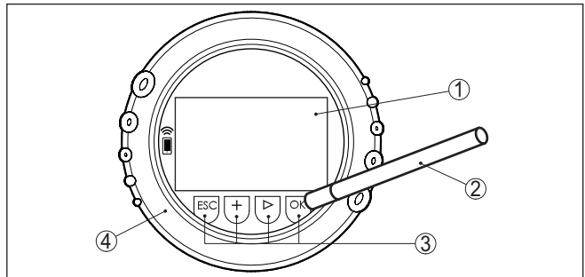
Fig. 51: Elementos de indicación y ajuste - con manejo mediante lápiz magnético
