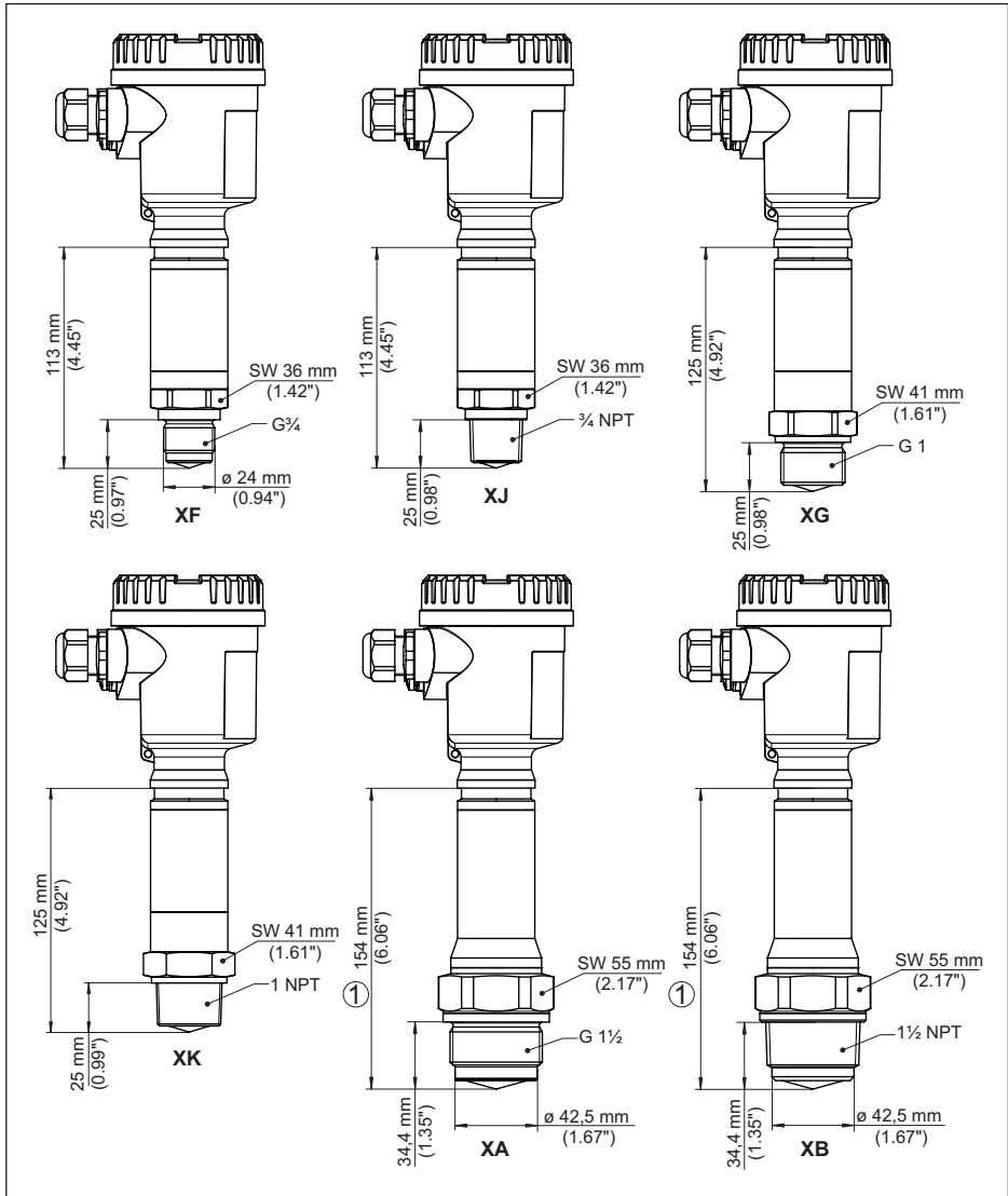
Fig. 85: NCR-86, rosca con sistema de antena integrado hasta +200 °C (+392 °F)/+250 °C (+482 °F)
