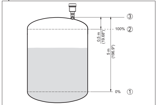
Fig. 52: Ejemplo de parametrización ajuste mín./máx. - Líquidos
