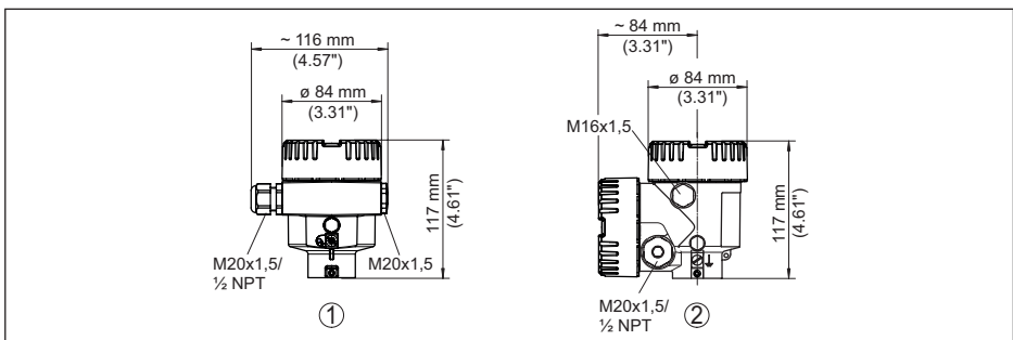
Fig. 76: Variantes de carcasa con tipo de protección IP66/IP68 (0,2 bar), (con el módulo de visualización y configuración montado aumenta la altura de la carcasa en 18 mm/0.71 in)
