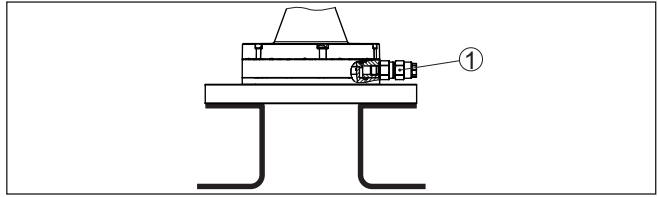
Fig. 39: Antena de trompeta de plástico con brida adaptadora 1 Conexión de aire de soplado
