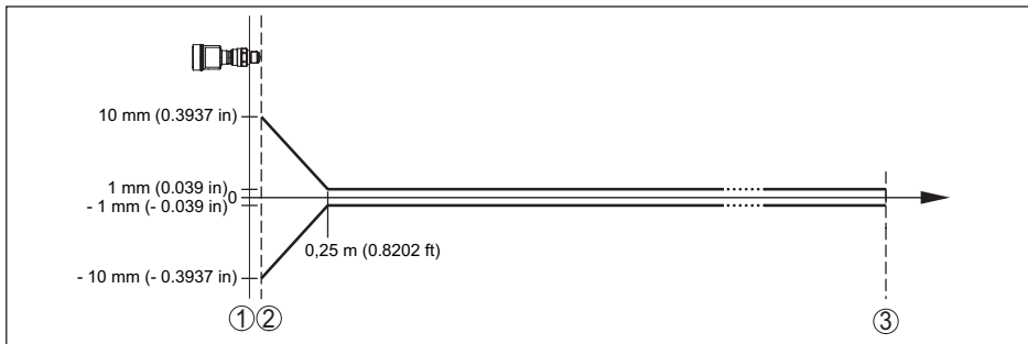
Fig. 59: Desviación de medición bajo condiciones de referencia (ejemplo rosca con sistema de antena integrado, vale correspondientemente para todas las versiones) 22)
