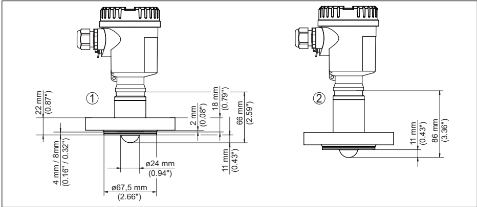
Fig. 89: NCR-86, sistema de antena encapsulado DN 25 PN 40
