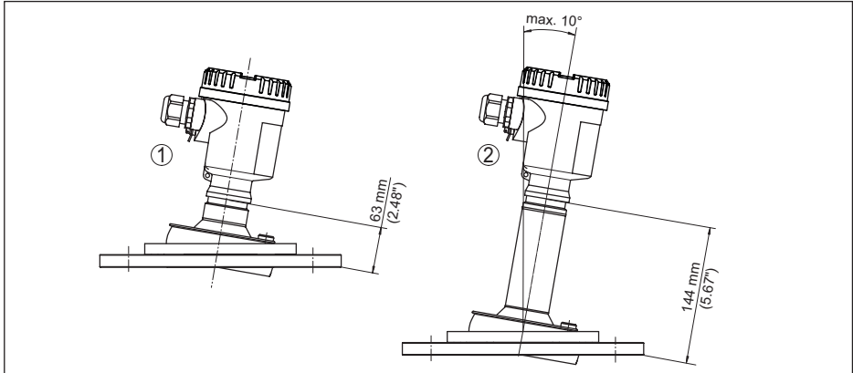
Fig. 96: NCR-86, brida con antena de lente y soporte giratorio
