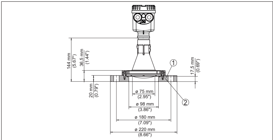
Fig. 80: NCR-86 con brida adaptadora DN 100 PN 6
