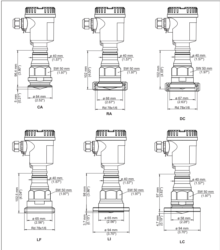
Fig. 92: NCR-86, conexión aséptica
