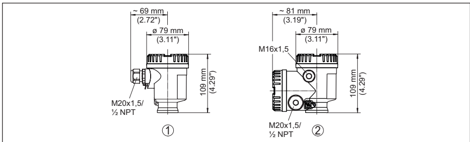
Fig. 75: Variantes de carcasa en grado de protección IP66/IP67; 1 bar (con módulo de visualización y configuración integrado aumenta la altura de la carcasa en 9 mm/0.35 in)
