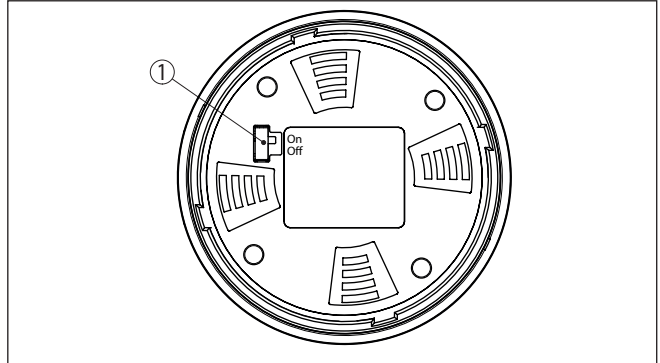
Fig. 54: Activar Bluetooth
