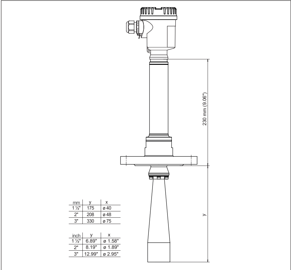
Fig. 88: NCR-86, brida con antena de trompeta versión 450 °C
