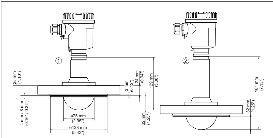
Fig. 90: NCR-86, sistema de antena encapsulado DN 80 PN 40
