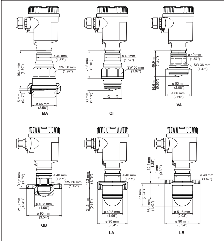
Fig. 93: NCR-86, conexión aséptica
