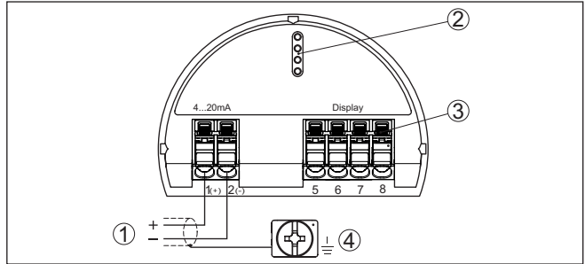
Fig. 45: Compartimento de la electrónica y de conexiones - Carcasa de una cámara
