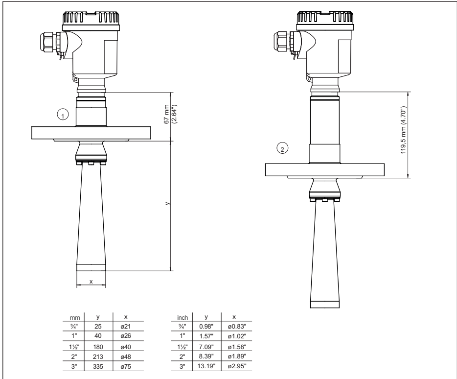
Fig. 86: NCR-86, brida con antena de trompeta hasta +150 °C (+302 °F)/+250 °C (+482 °F)
