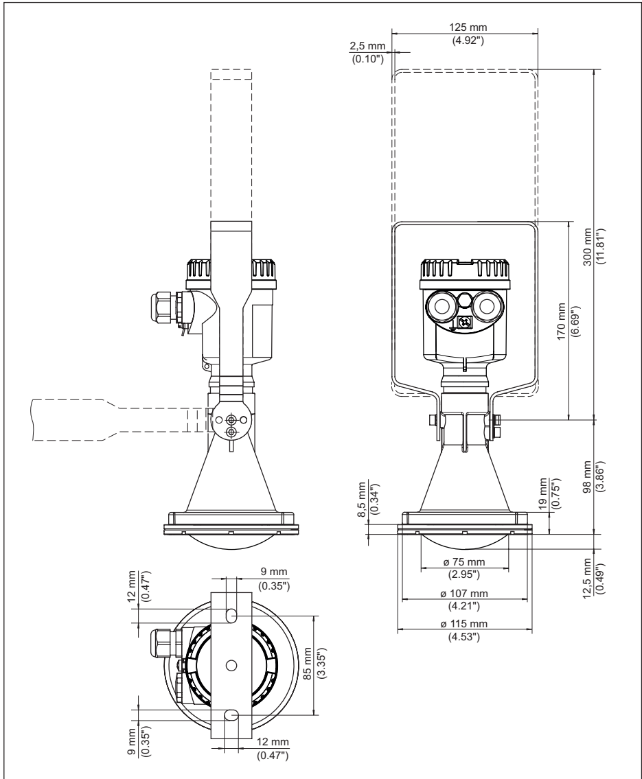
Fig. 82: NCR-86, antena de trompeta plástica, soporte de montaje con longitud de 170 ó 300 mm
