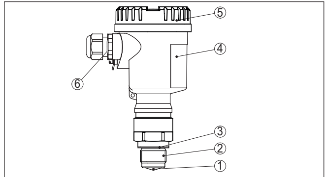
Fig. 1: Componentes del NCR-86
