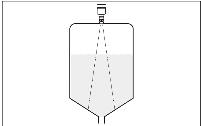
Fig. 17: Montaje del sensor de radar en depósito con fondo cónico
