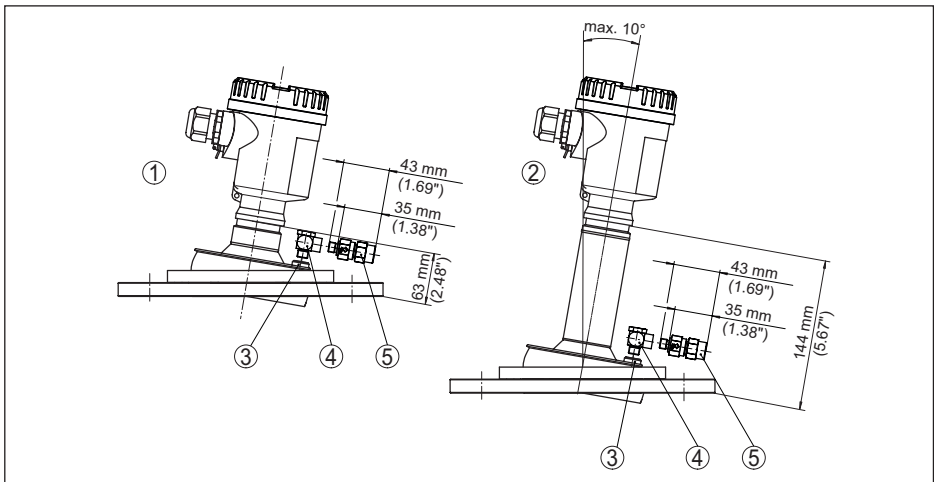
Fig. 97: NCR-86, brida con antena de lente, soporte giratorio y conexión de aire de soplado
