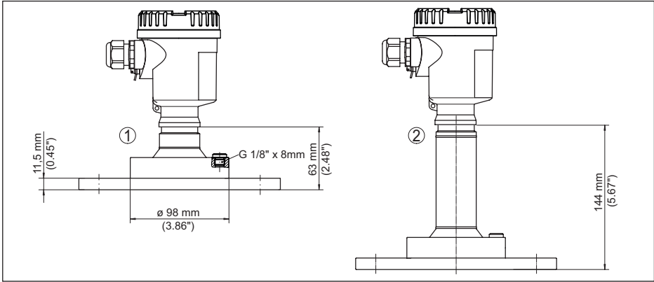
Fig. 94: NCR-86, brida con antena de lente (ver dibujo para el grosor de la brida, dimensiones de la brida según DIN, ASME, JIS)
