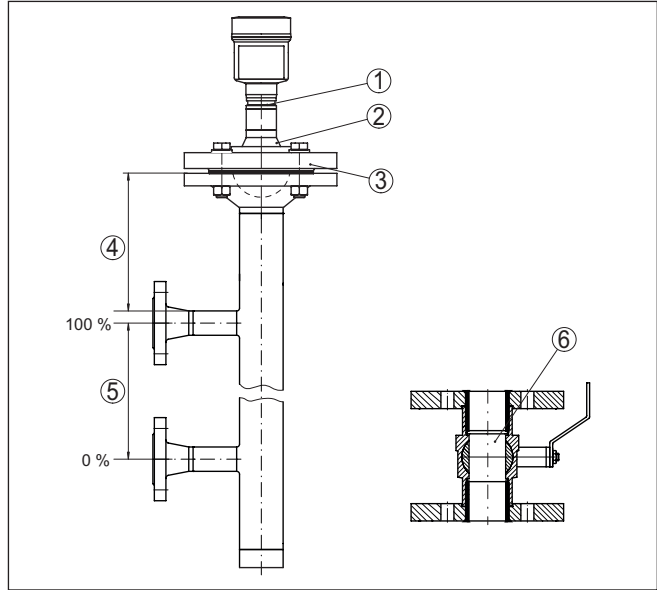
Fig. 41: Montaje bypass
