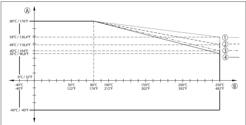
Fig. 63: Reducción de temperatura ambiente, rosca G1½ con sistema de antena integrada hasta +250 °C (+482 °F)
