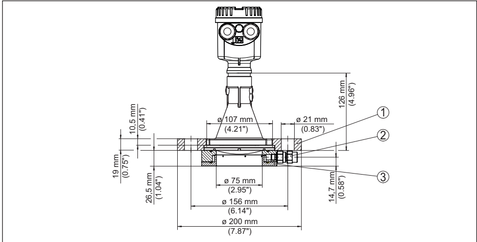
Fig. 79: NCR-86 con brida de compresión y conexión de purga aire adecuada para 3" 150 lbs, DN 80 PN 16
