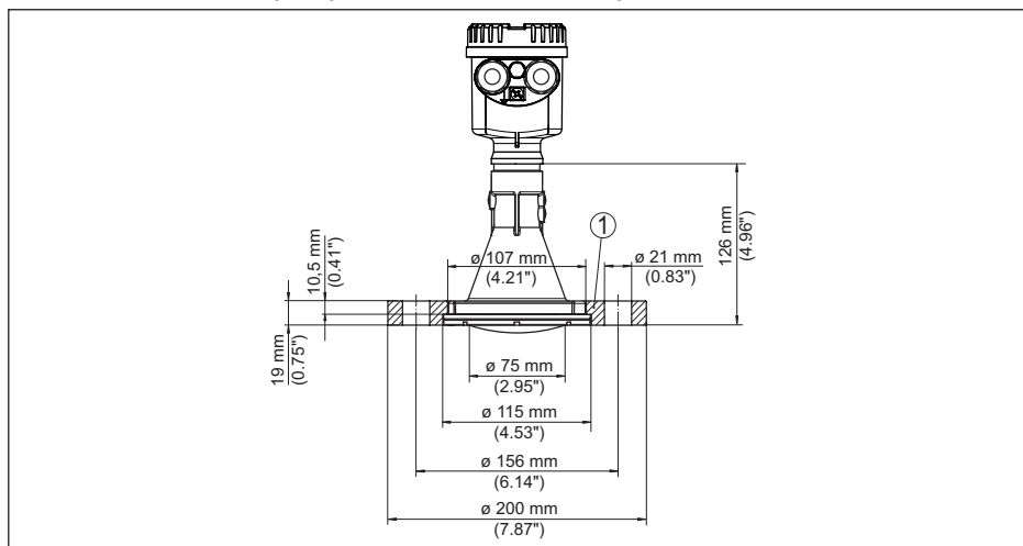
Fig. 78: NCR-86 con brida de compresión adecuada para 3" 150 lbs, DN 80 PN 16
