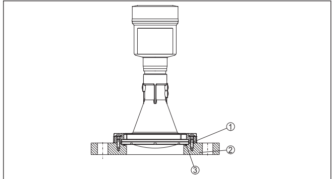
Fig. 14: Brida adaptadora
