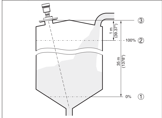
Fig. 53: Ejemplo de parametrización ajuste mín./máx. - Sólidos a granel
