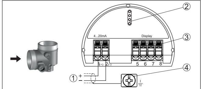
Fig. 47: Compartimiento de conexiones - Carcasa de dos cámaras
