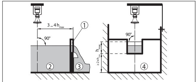
Fig. 42: Medición de caudal con canal rectangular: h_{\text{máx.}} = llenado máx. del canal rectangular
