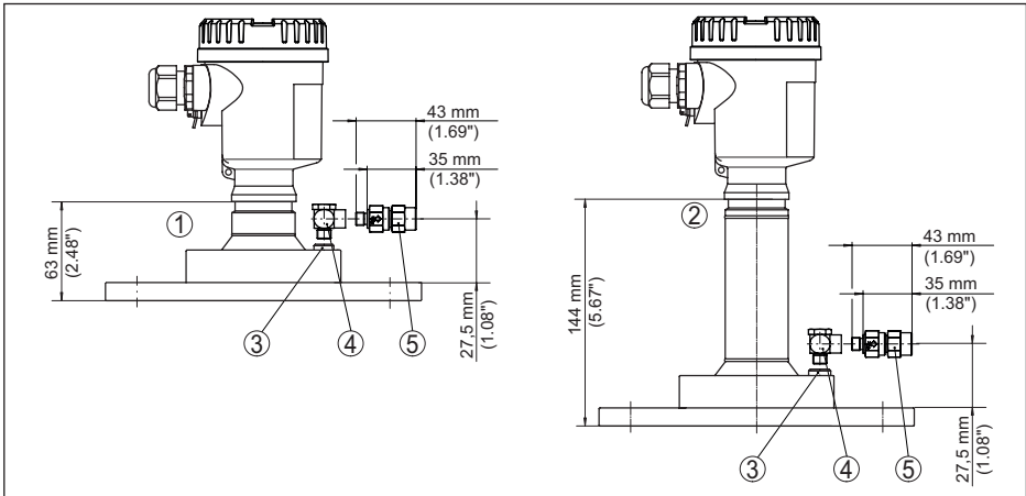
Fig. 95: NCR-86, Brida con antena de lente y conexión de aire de soplado
