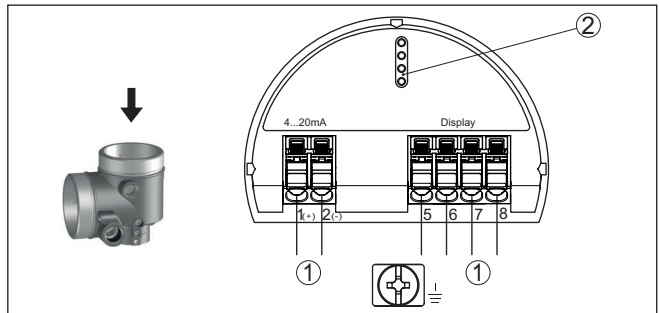
Fig. 46: Compartimiento de la electrónica - Carcasa de dos cámaras.
