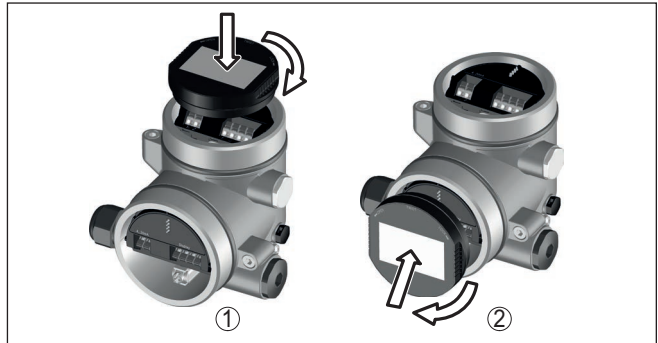
Fig. 49: Empleo del módulo de visualización y configuración en carcasa de dos cámaras
