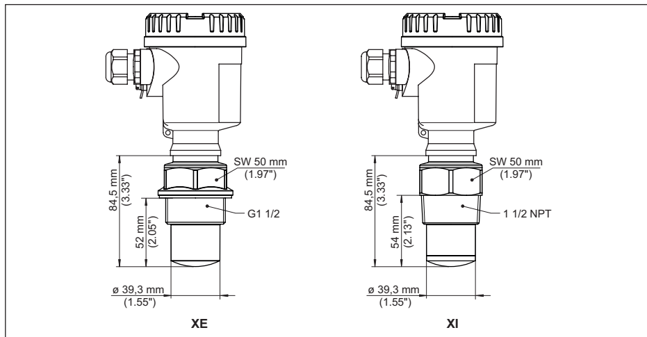
Fig. 83: NCR-86, rosca con sistema de antena integrado hasta +80 °C (+176 °F)
