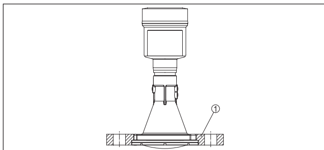
Fig. 12: Brida de compresión universal
