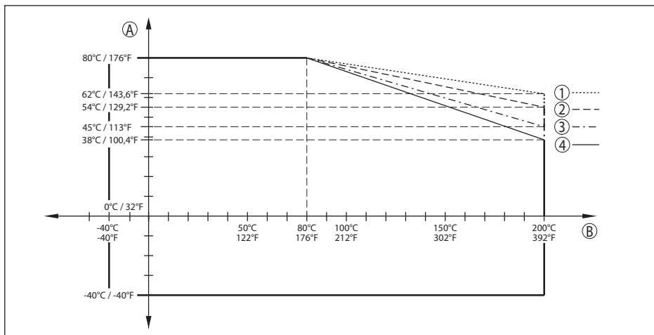
Fig. 63: Reducción de temperatura ambiente, brida con sistema de antena encapsulado hasta +200 °C (+392 °F)
