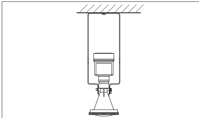
Fig. 9: Montaje en el techo mediante el estribo de montaje con una longitud de 300 mm
