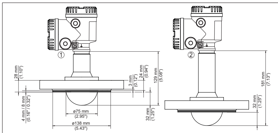
Fig. 85: NCR-86, sistema de antena encapsulado DN 80 PN 40
