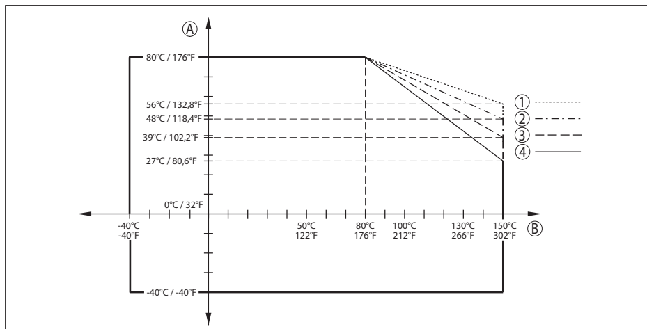
Fig. 68: Derating temperatura ambiente, conexión higiénica hasta +150 °C (+302 °F)
