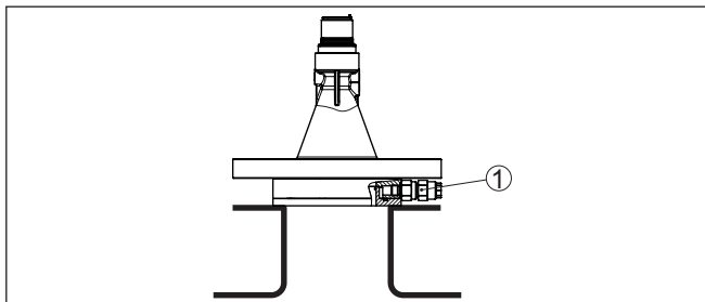
Fig. 37: Antena de trompeta plástica con brida de compresión
