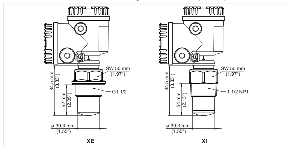
Fig. 78: NCR-86, rosca con sistema de antena integrado hasta +80 °C (+176 °F)
