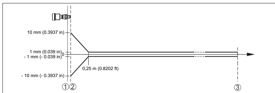
Fig. 56: Desviación de medición bajo condiciones de referencia (ejemplo rosca con sistema de antena integrado, vale correspondientemente para todas las versiones) 22)
