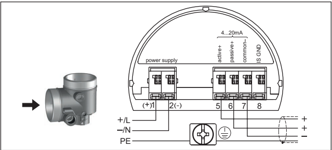
Fig. 45: Compartimiento de conexiones carcasa de dos cámaras con tensión de red
