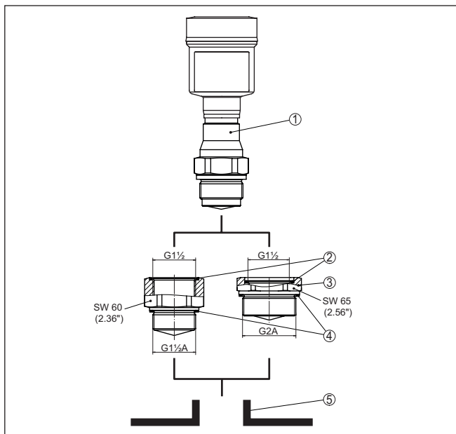
Fig. 26: NCR-86 con adaptador de rosca PTFE (ejemplo NCR-86 con rosca G1½)
