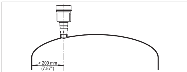
Fig. 15: Montaje del sensor en tapas de depósito redondas
