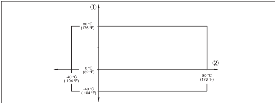
Fig. 57: Reducción de temperatura ambiente, antena de trompeta plástica
