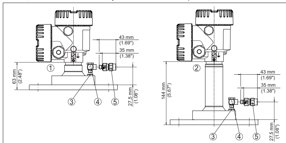
Fig. 90: NCR-86, Brida con antena de lente y conexión de aire de soplado
