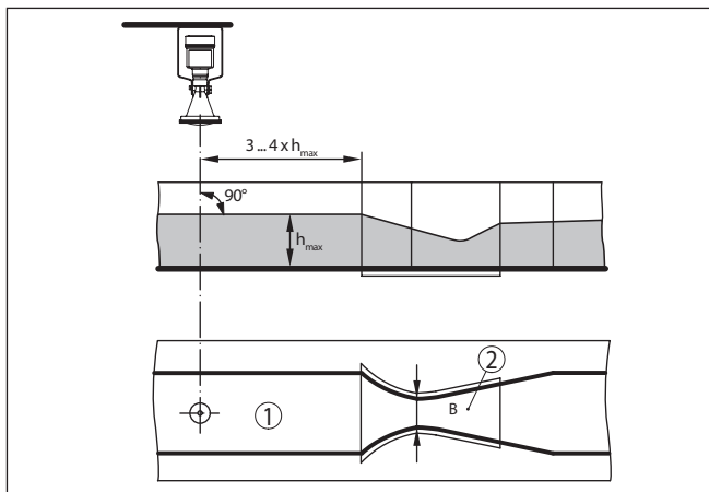
Fig. 42: Medición de caudal con canal venturi Khafagi: h_{\max} = llenado máx. del canal; B = mayor estrechamiento del canal
