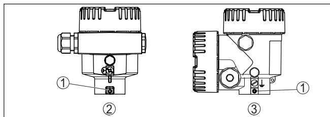
Fig. 4: Posición del tornillo de bloqueo según la carcasa
