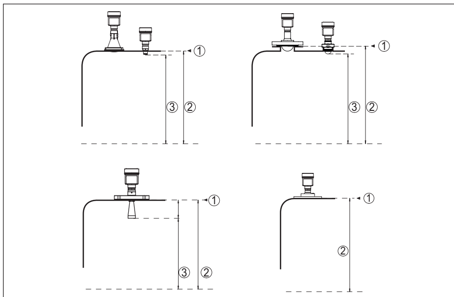
Fig. 55: Datos para la magnitud de entrada
