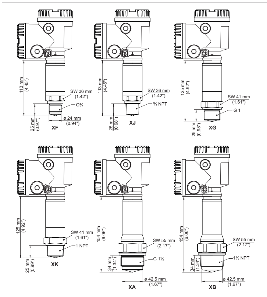
Fig. 80: NCR-86, rosca con sistema de antena integrado hasta +200 °C (+392 °F) y +250 °C (+482 °F)
