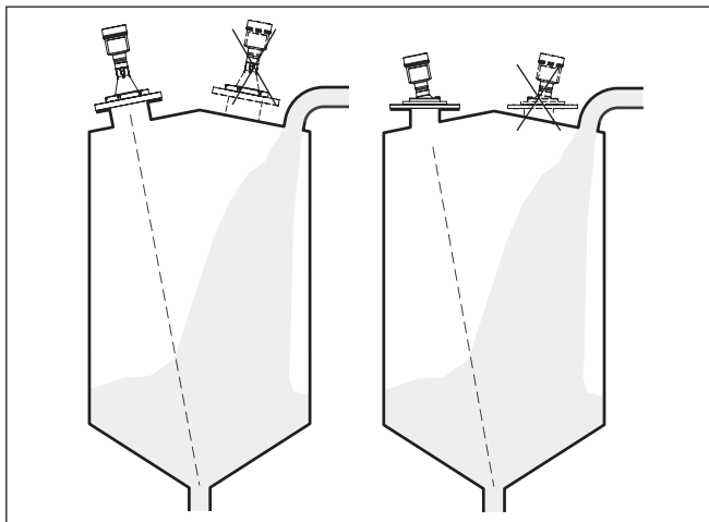
Fig. 20: Montaje del sensor de radar con entrada de producto – llenado por arriba
