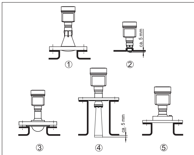
Fig. 22: Montaje en tubuladura recomendado con diferentes versiones del NCR-86
