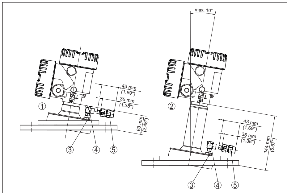
Fig. 92: NCR-86, brida con antena de lente, soporte giratorio y conexión de aire de soplado
