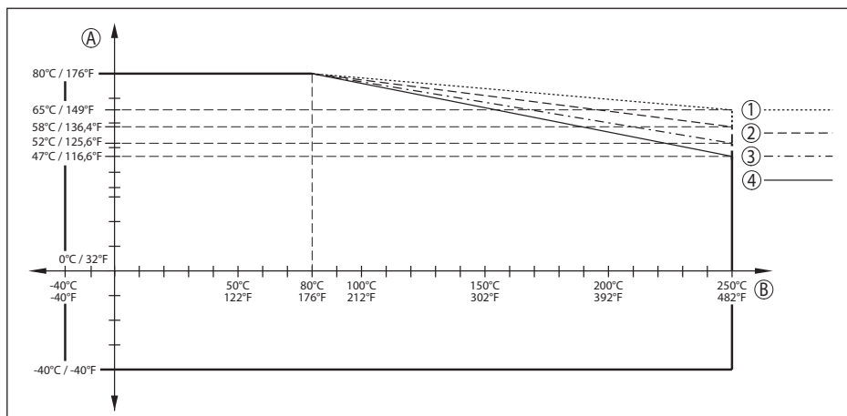
Fig. 67: Reducción de temperatura ambiente, brida con antena de lente hasta +250 °C (+482 °F)
