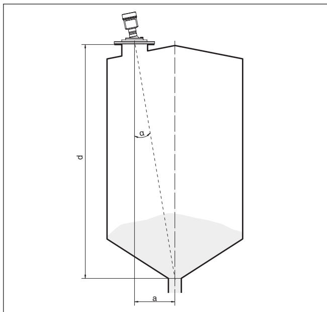
Fig. 31: Determinación del ángulo de inclinación para la alineación del NCR-86
