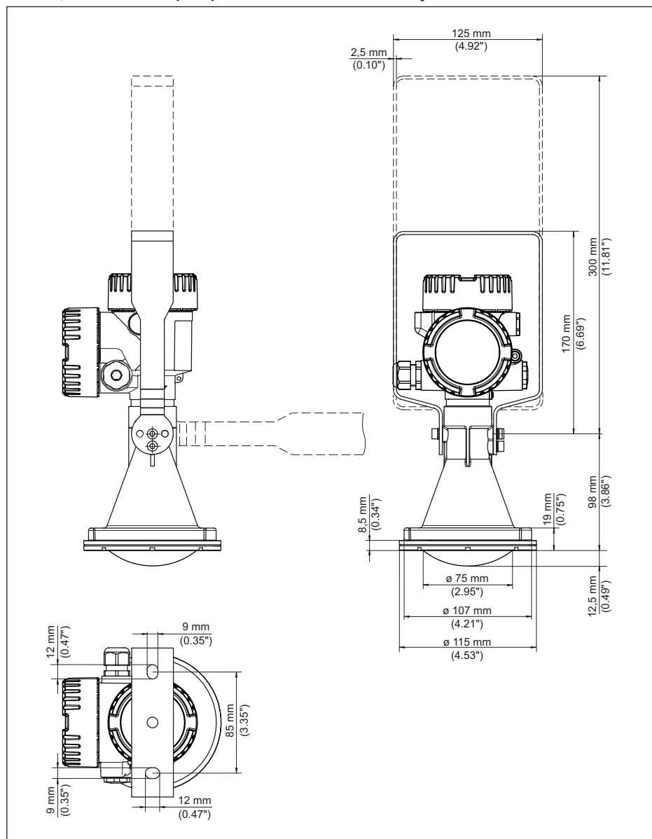
Fig. 77: NCR-86, antena de trompeta plástica, soporte de montaje con longitud de 170 ó 300 mm
