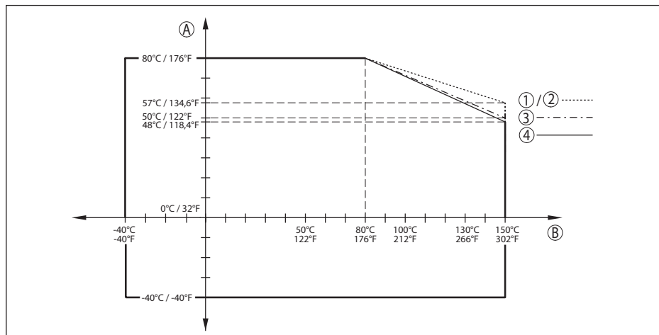
Fig. 61: Reducción de temperatura ambiente, brida con sistema de antena encapsulado hasta +150 °C (+302 °F)
