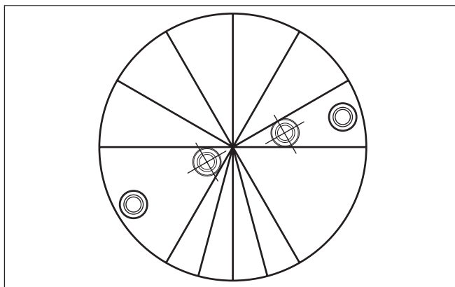
Fig. 35: Montaje e instalación en silos de varias cámaras
