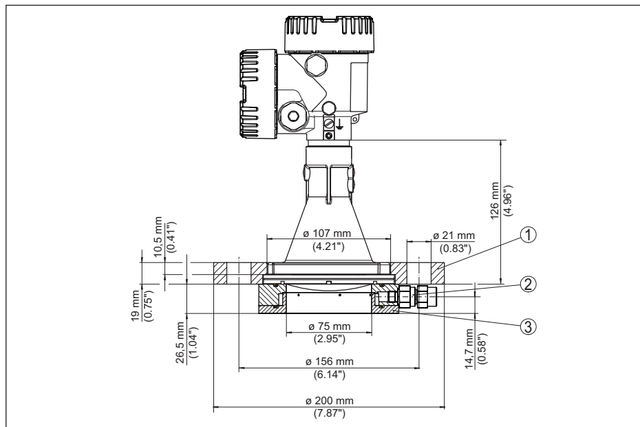
Fig. 74: NCR-86 con brida de compresión y conexión de purga aire adecuada para 3" 150 lbs, DN 80 PN 16
