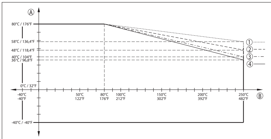
Fig. 60: Reducción de temperatura ambiente, rosca G1½ con sistema de antena integrada hasta +250 °C (+482 °F)
