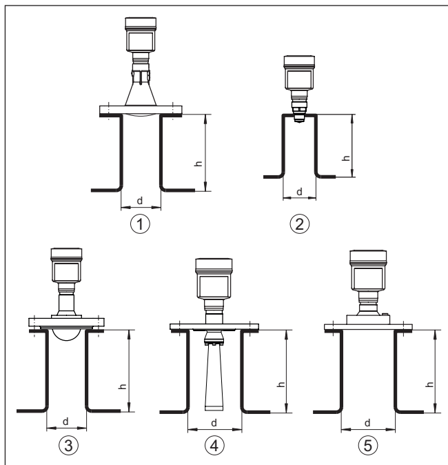
Fig. 23: Montaje en tubuladura recomendado en caso de dimensiones de tubuladura divergentes con diferentes versiones del NCR-86
