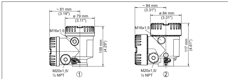
Fig. 72: NCR-86: con módulo de visualización y configuración integrado aumenta la altura de la carcasa en 9 mm (0.35 in)
