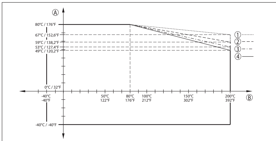
Fig. 59: Reducción de temperatura ambiente, rosca G1½ con sistema de antena integrada hasta +200 °C (+392 °F)
