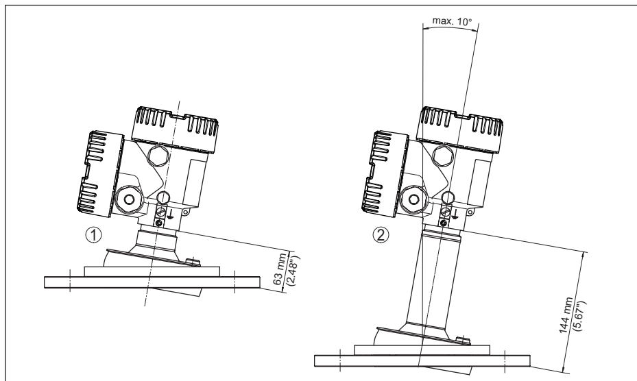
Fig. 91: NCR-86, brida con antena de lente y soporte giratorio
