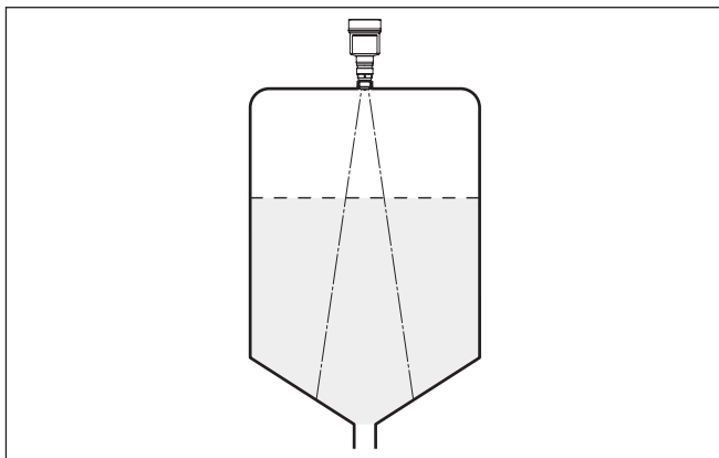
Fig. 16: Montaje del sensor de radar en depósito con fondo cónico
