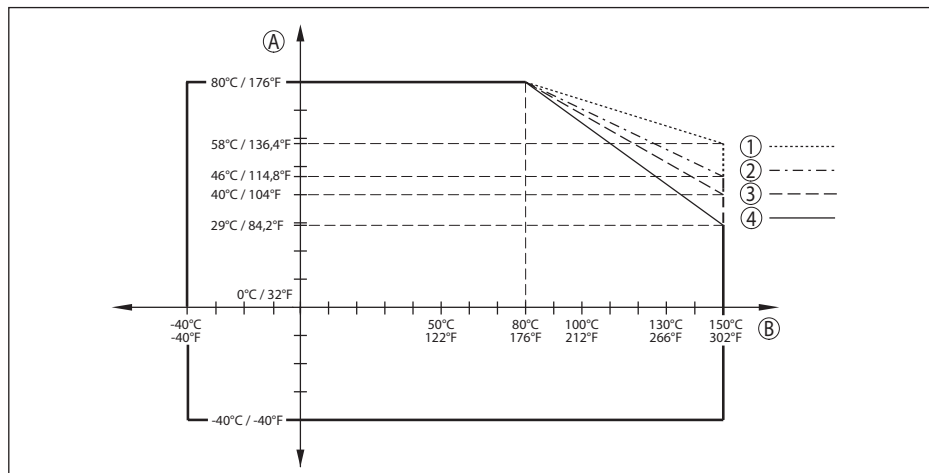
Fig. 58: Reducción de temperatura ambiente, rosca G1½ con sistema de antena integrada hasta +150 °C (+302 °F)
