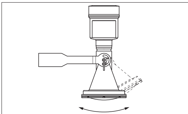
Fig. 7: Ajuste de la inclinación durante el montaje horizontalmente en la pared
