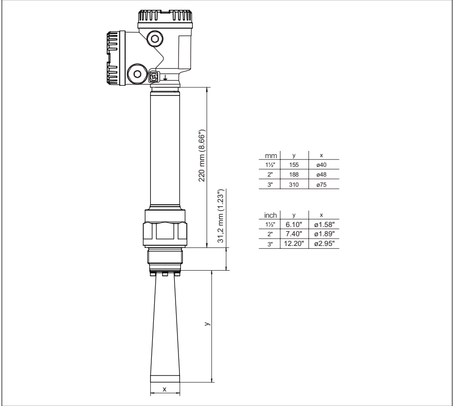
Fig. 82: NCR-86, rosca con antena de trompeta versión 450 °C
