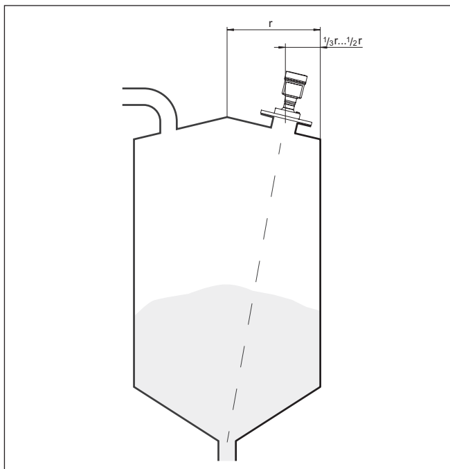
Fig. 30: Posición de montaje y alineación
