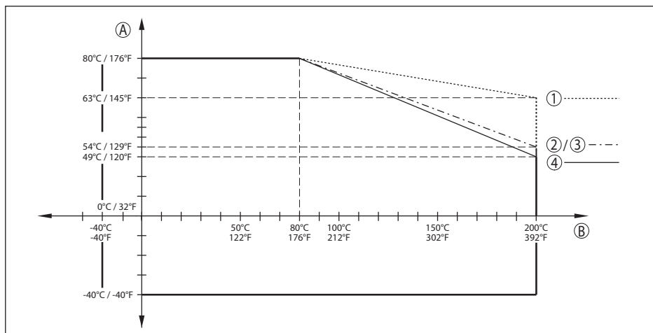
Fig. 66: Reducción de temperatura ambiente, brida con antena de lente hasta +200 °C (+392 °F)
