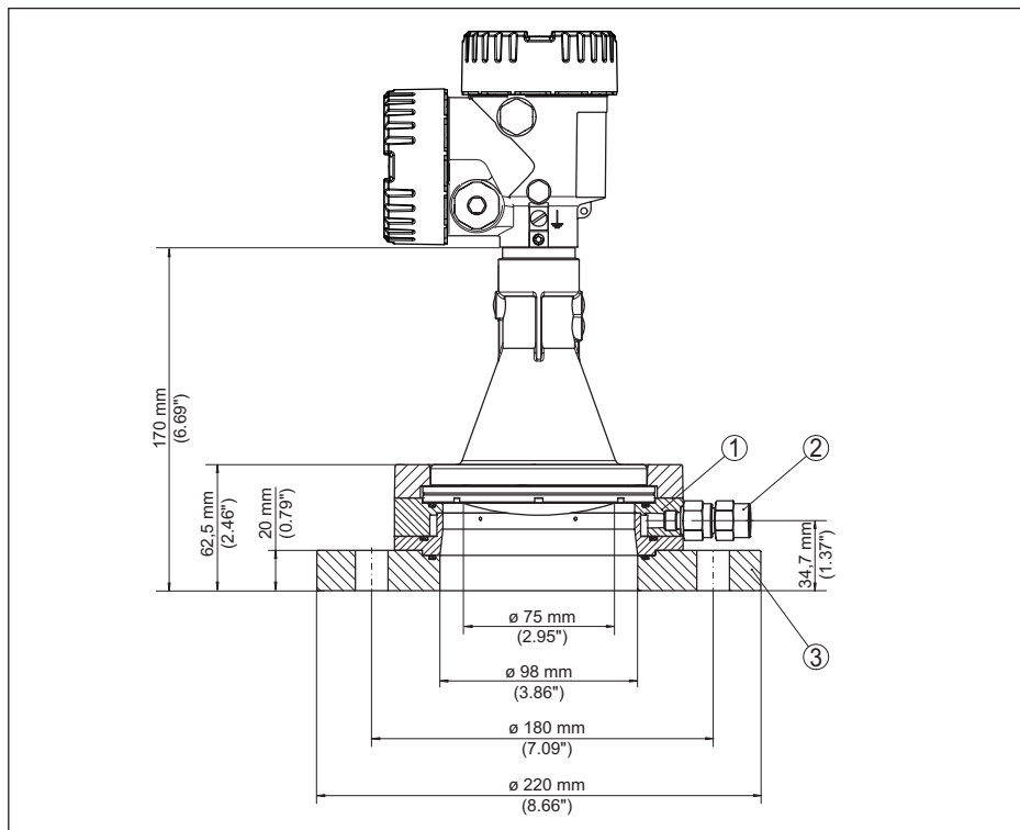
Fig. 76: NCR-86, brida adaptadora y conexión de aire de soplado DN 100 PN 6
