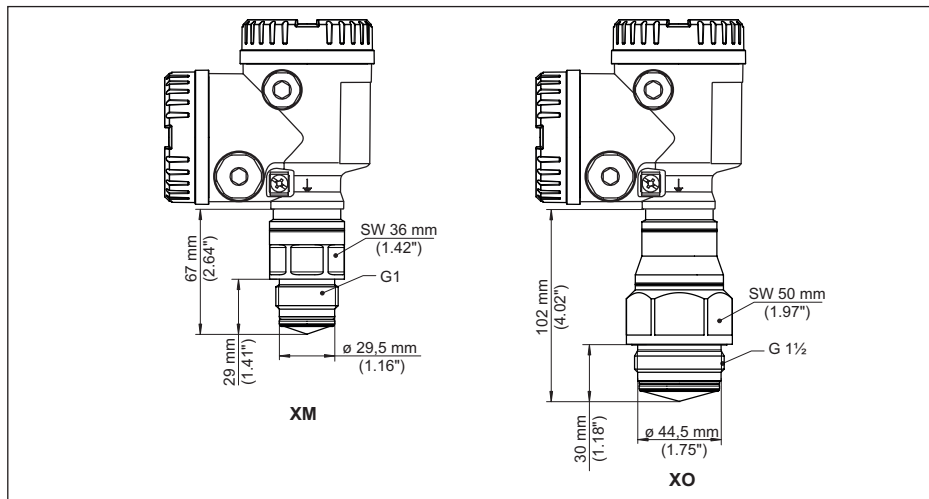
Fig. 86: NCR-86, rosca para adaptador higiénico
