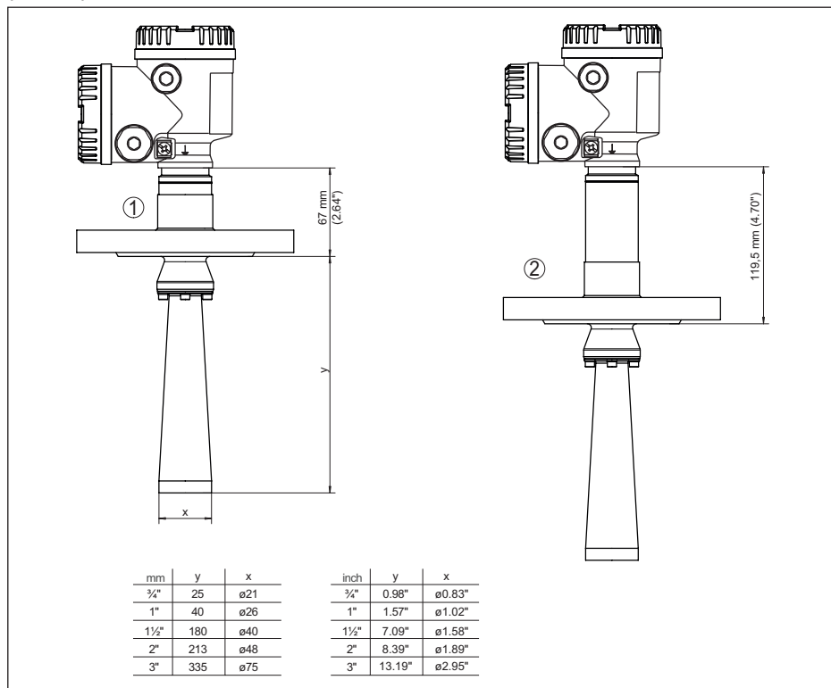
Fig. 81: NCR-86, brida con antena de trompeta hasta +150 °C (+302 °F)/+250 °C (+482 °F)
