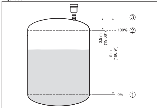
Fig. 49: Ejemplo de parametrización ajuste mín./máx. - Líquidos
