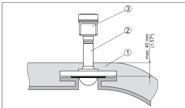
Fig. 27: Montaje del equipo con depósitos aislados
