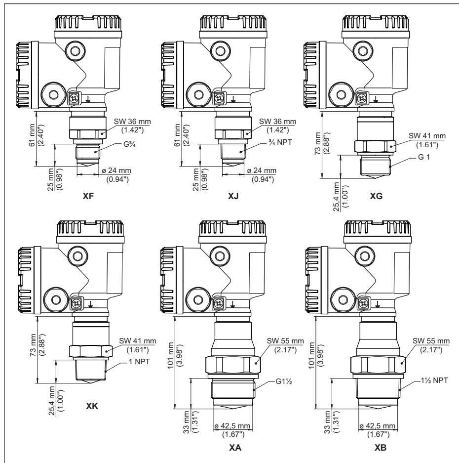
Fig. 79: NCR-86, rosca con sistema de antena integrado hasta +150 °C (+302 °F)
