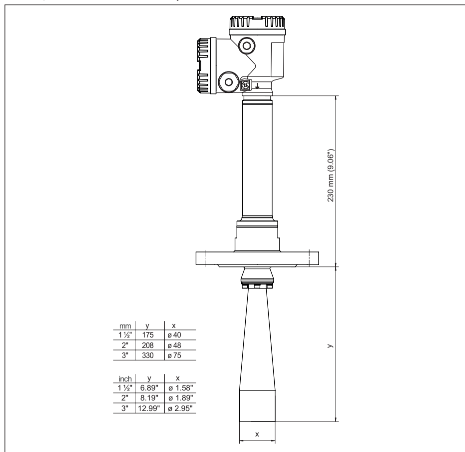
Fig. 83: NCR-86, brida con antena de trompeta versión 450 °C
