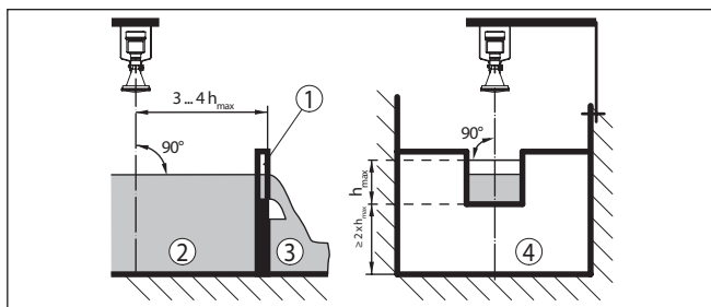
Fig. 41: Medición de caudal con canal rectangular: h_{\text{máx.}} = llenado máx. del canal rectangular
