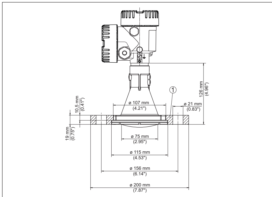
Fig. 73: NCR-86 con brida de compresión adecuada para 3" 150 lbs, DN 80 PN 16
