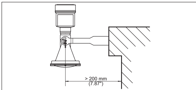
Fig. 10: Montaje en pared horizontal mediante el soporte de montaje con una longitud de 170 mm
