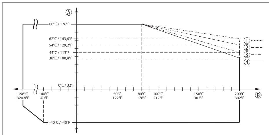
Fig. 64: Reducción de temperatura ambiente, brida con sistema de antena encapsulado -196 ... +200 °C (-320.8 ... +392 °F)
