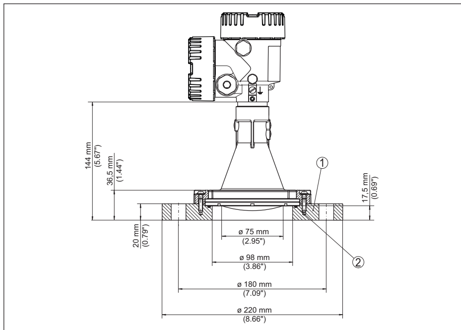
Fig. 75: NCR-86 con brida adaptadora DN 100 PN 6
