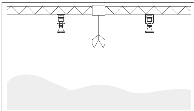
Fig. 34: Sensores de radar en la viga de una grúa
