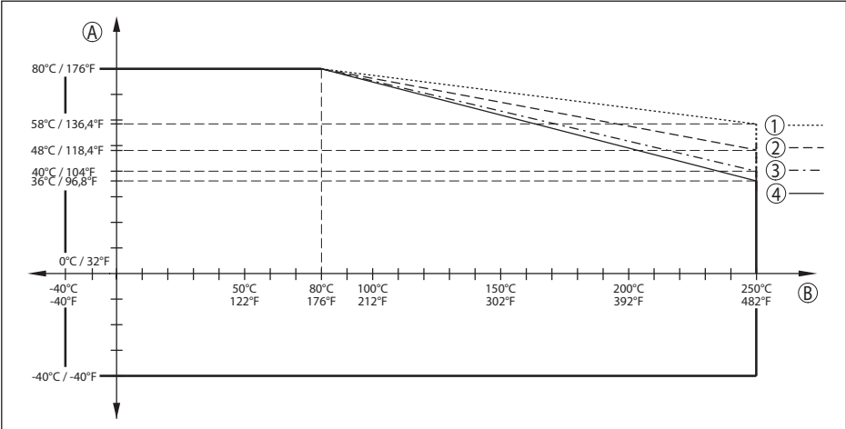
Fig. 71: Reducción de temperatura ambiente, brida con antena de trompeta hasta +250 °C (+482 °F)
