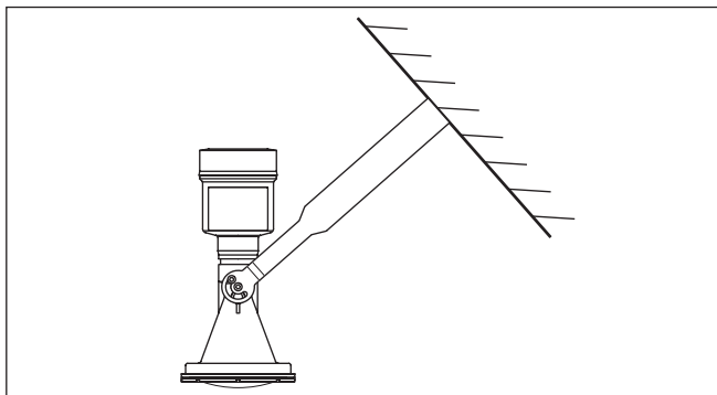
Fig. 11: Montaje en pared oblicua mediante el estribo de montaje con una longitud de 300 mm
