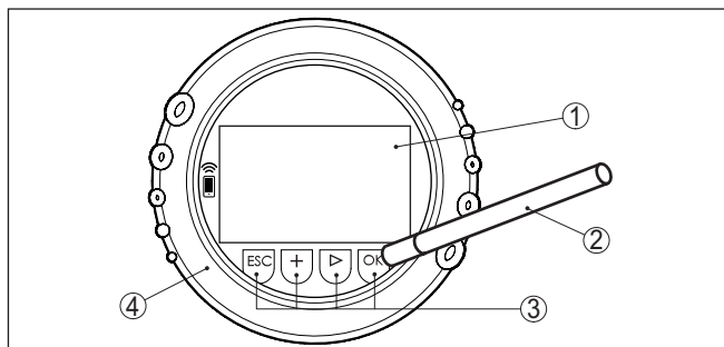
Fig. 48: Elementos de indicación y ajuste - con manejo mediante lápiz magnético
