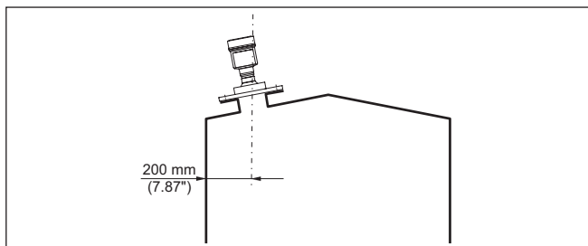
Fig. 17: Montaje del sensor en la tapa de depósito
