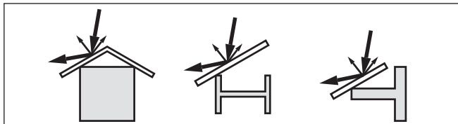
Fig. 28: Tapar los perfiles lisos con pantallas dispersoras
