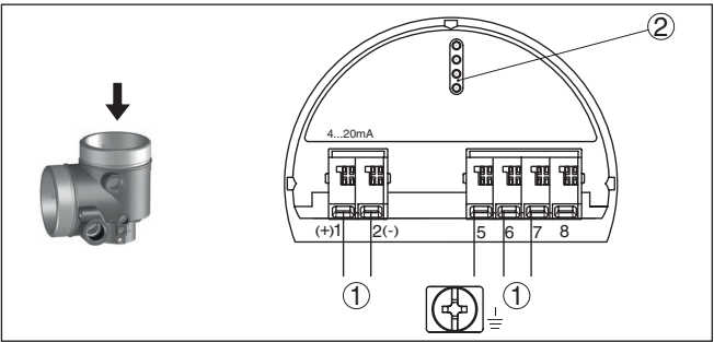
Fig. 44: Compartimiento de la electrónica - Carcasa de dos cámaras.
