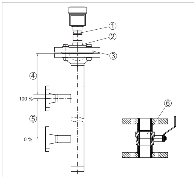
Fig. 40: Montaje bypass
