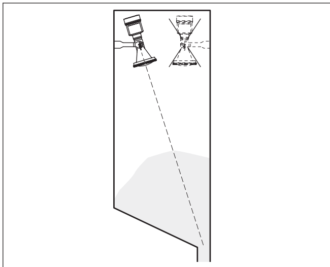
Fig. 36: Montaje e instalación en silos de varias cámaras
