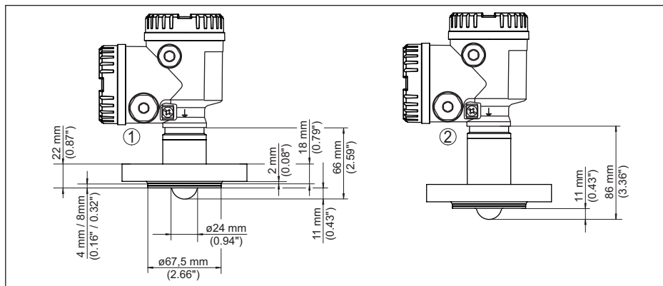
Fig. 84: NCR-86, sistema de antena encapsulado DN 25 PN 40
