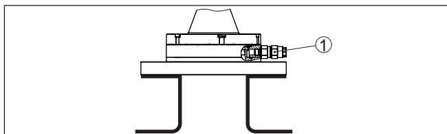
Fig. 38: Antena de trompeta de plástico con brida adaptadora
