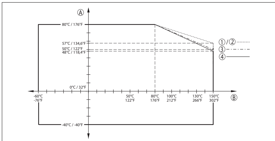
Fig. 62: Reducción de temperatura ambiente, brida con sistema de antena encapsulado -60 ... +150 °C (-76 ... +302 °F)
