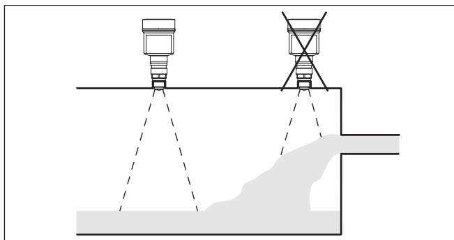
Fig. 19: Montaje del sensor de radar en flujo de entrada de producto
