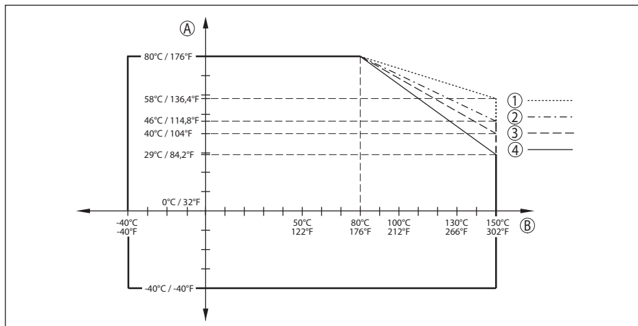
Fig. 69: Reducción de temperatura ambiente, brida con antena de trompeta hasta +150 °C (+302 °F)
