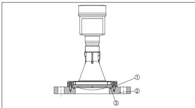
Fig. 13: Brida adaptadora
