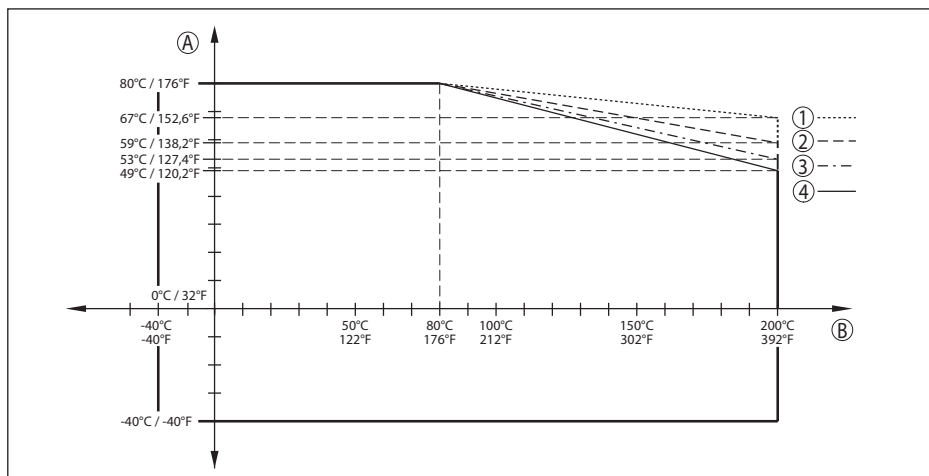
Fig. 70: Reducción de temperatura ambiente, brida con antena de trompeta hasta +200 °C (+392 °F)
