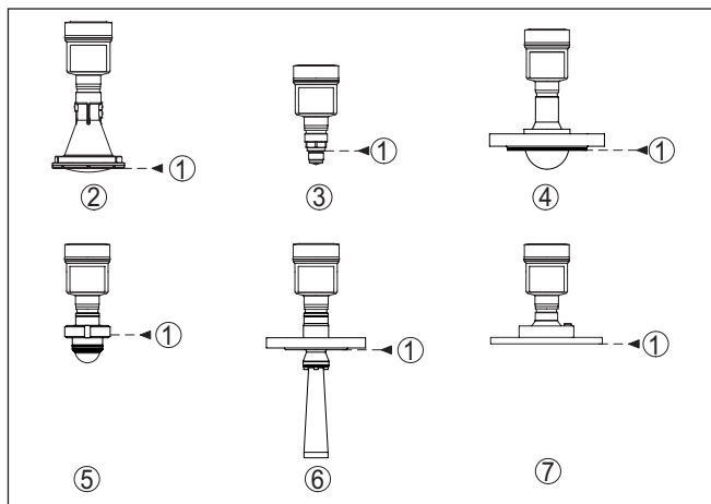
Fig. 18: Posición del plano de referencia
