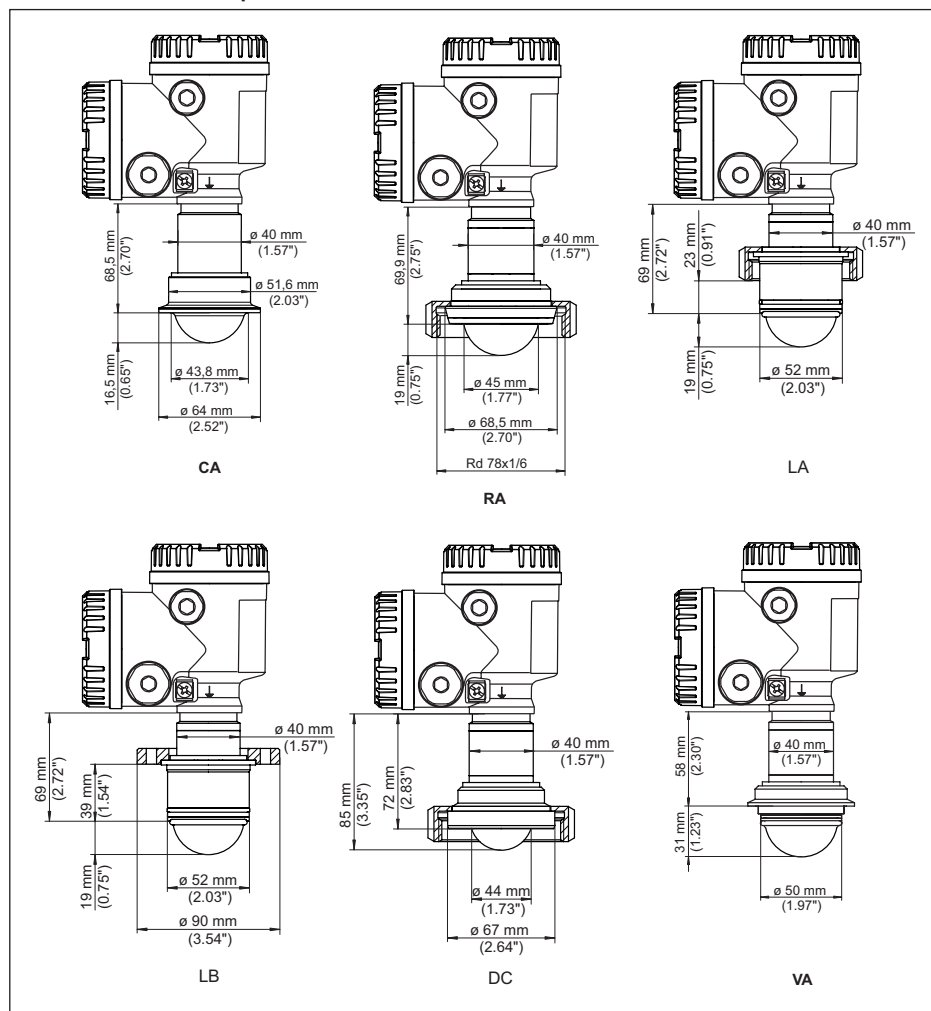
Fig. 87: NCR-86, conexión aséptica
