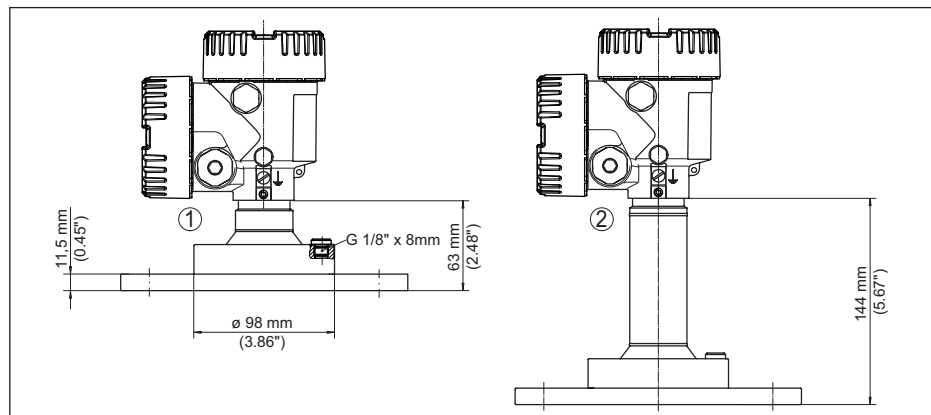
Fig. 89: NCR-86, brida con antena de lente (ver dibujo para el grosor de la brida, dimensiones de la brida según DIN, ASME, JIS)
