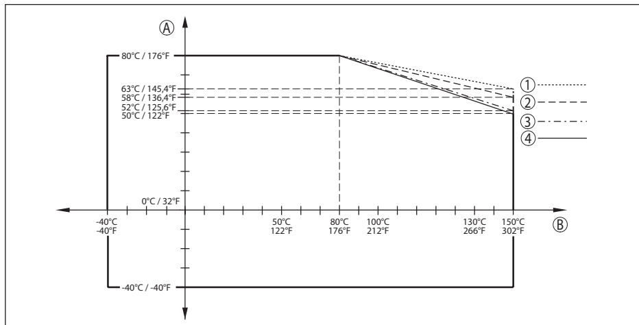
Fig. 65: Reducción de temperatura ambiente, brida con antena de lente hasta +150 °C (+302 °F)
