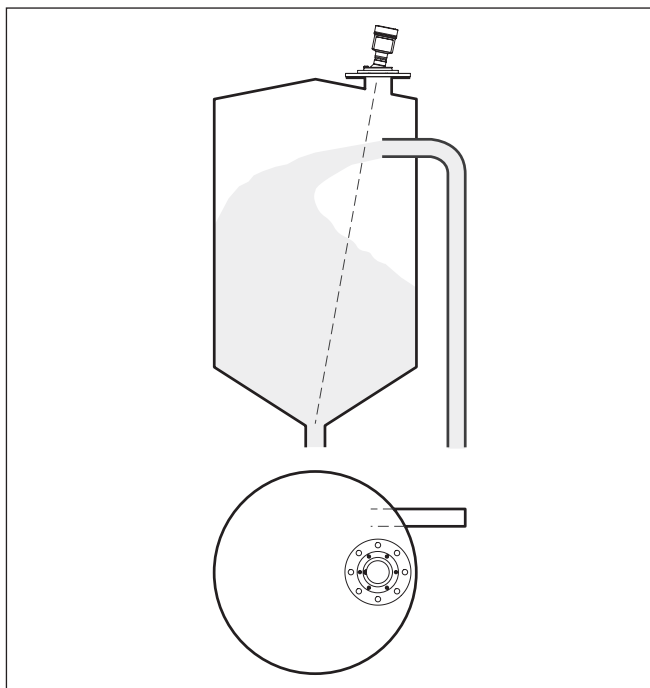
Fig. 21: Montaje del sensor de radar con entrada de producto – llenado lateral
