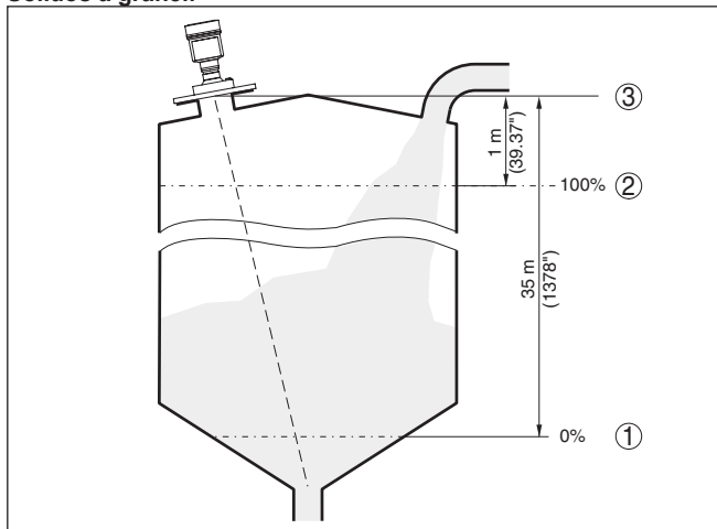
Fig. 50: Ejemplo de parametrización ajuste mín./máx. - Sólidos a granel
