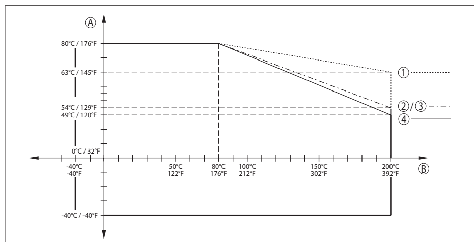
Fig. 69: Derating température ambiante, bride avec antenne lentille jusqu'à +200 °C (+392 °F)
