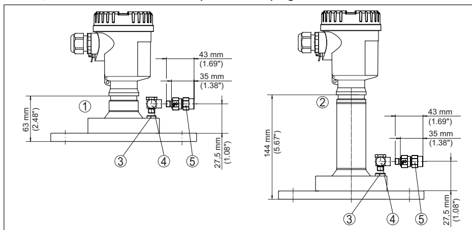
Fig. 95: NCR-86, bride avec antenne lentille et prise d'air de purge
