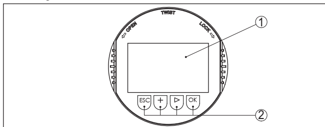
Fig. 50: Éléments de réglage et d'affichage
