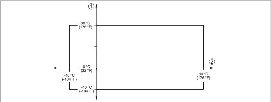
Fig. 60: Derating température ambiante, antenne cône en plastique
