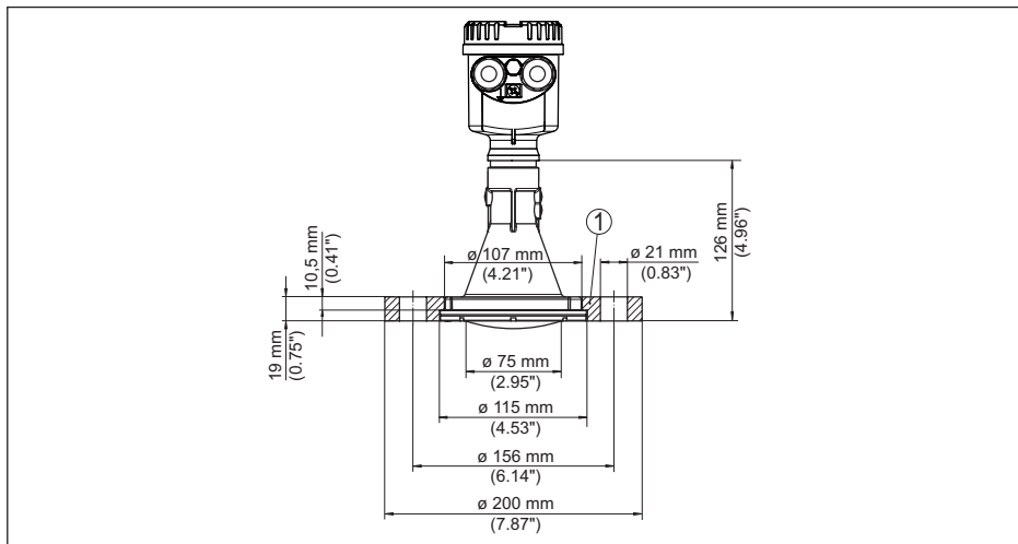
Fig. 78: NCR-86 avec bride tournante convenant à la bride 3" 150 lbs, DN 80 PN 16
