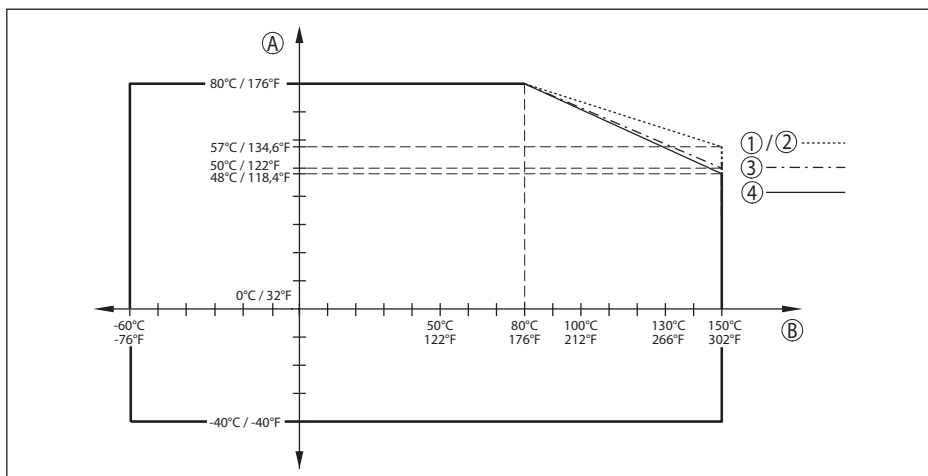
Fig. 65: Derating température ambiante, bride avec système d'antenne encapsulé -60 ... +150 °C (-76 ... +302 °F)
