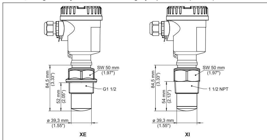
Fig. 83: NCR-86, filetage avec système d'antenne intégré jusqu'à +80 °C (+176 °F)
