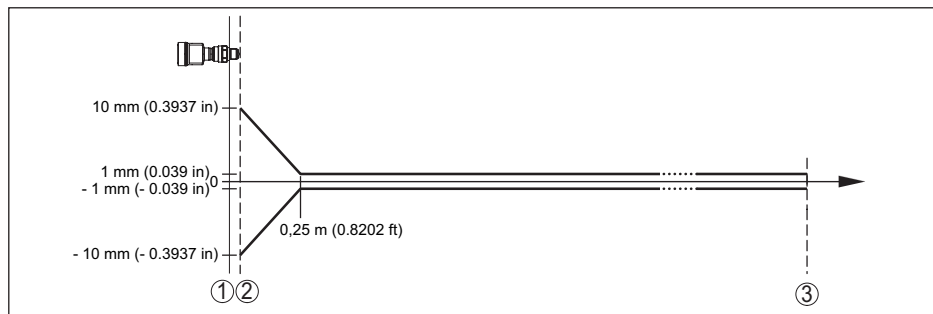
Fig. 59: Écart de mesure sous les conditions de référence (exemple filetage avec système d'antenne intégré, s'applique en conséquence pour toutes les versions) 22)
