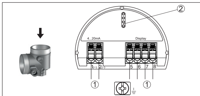
Fig. 46: Compartiment électronique - boîtier à deux chambres
