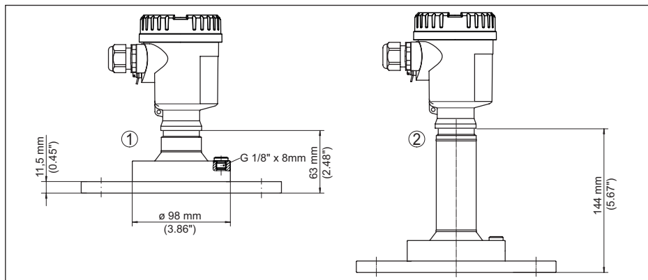
Fig. 94: NCR-86, bride avec antenne lentille (épaisseur de la bride cf. schéma, cote de la bride selon DIN, ASME, JIS)
