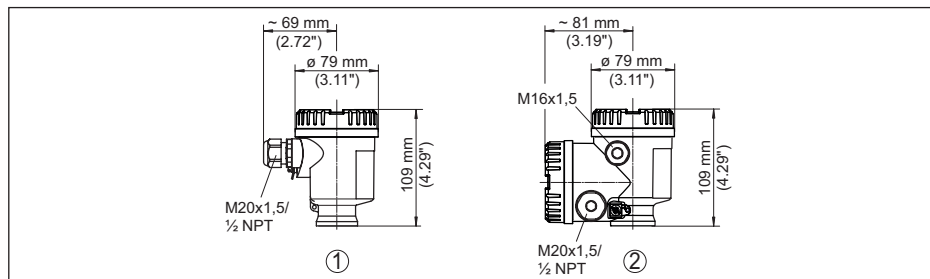
Fig. 75: Variantes de boîtier en protection IP66/IP67 (avec un module de réglage et d'affichage intégré, la hauteur du boîtier augmente de 9 mm/0.35 in)
