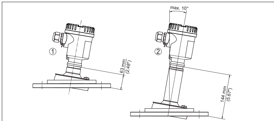
Fig. 96: NCR-86, bride avec antenne lentille et rotule d'orientation
