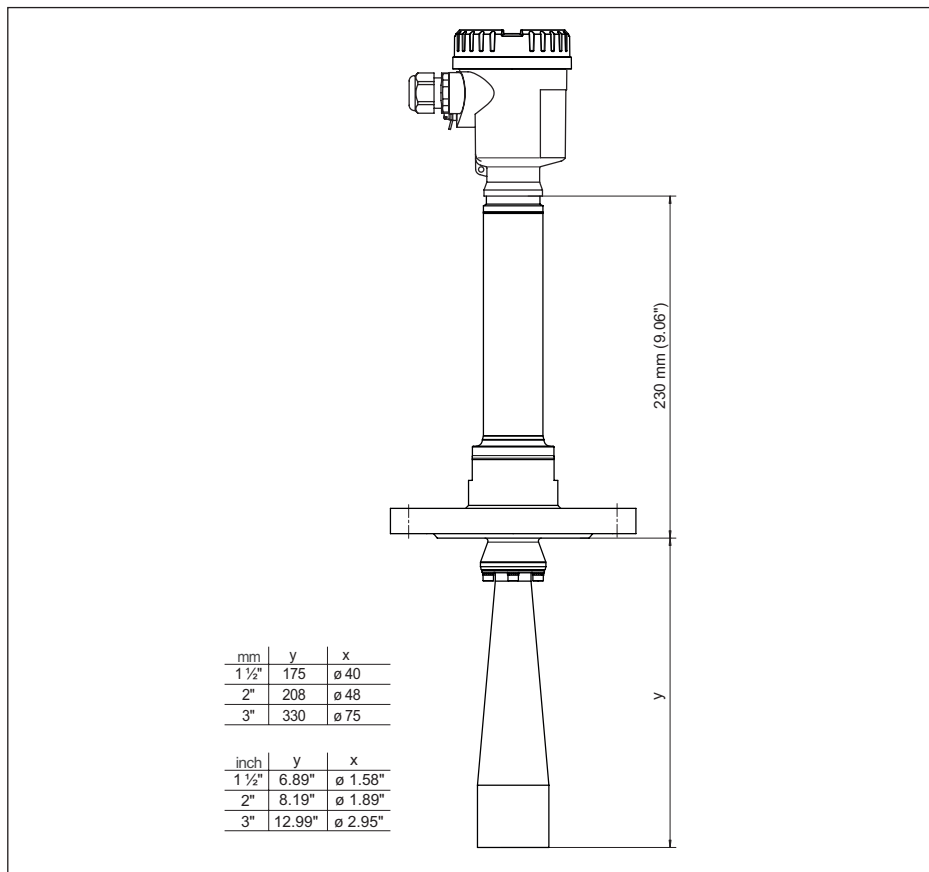
Fig. 88: NCR-86, bride avec antenne cône version 450 °C
