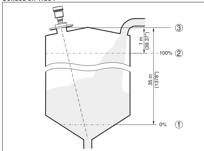
Fig. 53: Exemple de paramétrage du réglage min./max. - Solides en vrac
