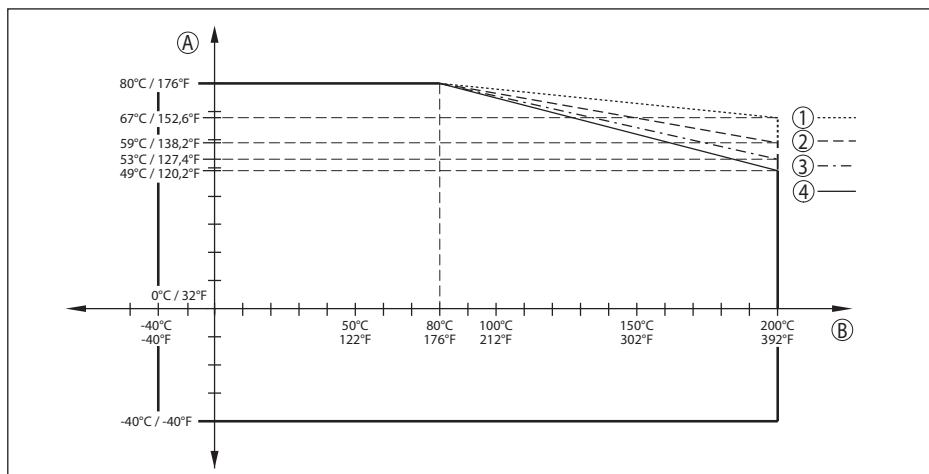
Fig. 73: Derating température ambiante, bride avec antenne cône jusqu'à +200 °C (+392 °F)
