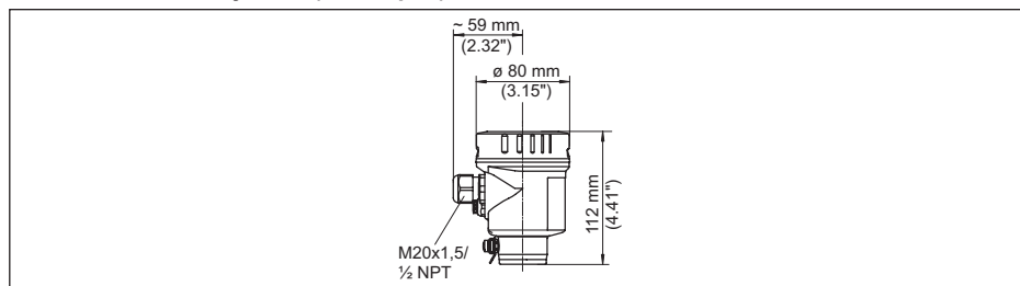
Fig. 77: Variantes de boîtier en protection IP66/IP68 (0,2 bar), (avec un module de réglage et d'affichage intégré, la hauteur du boîtier augmente de 18 mm/0.71 in)
