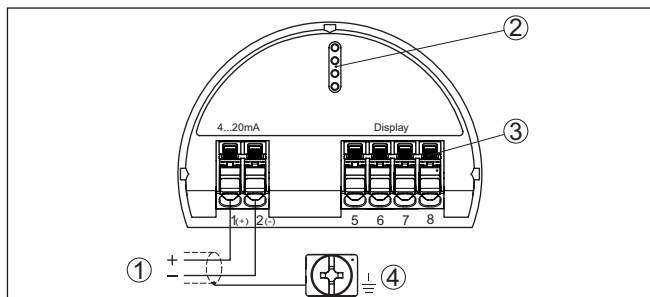
Fig. 45: Compartiment électronique et de raccordement - boîtier à chambre unique
