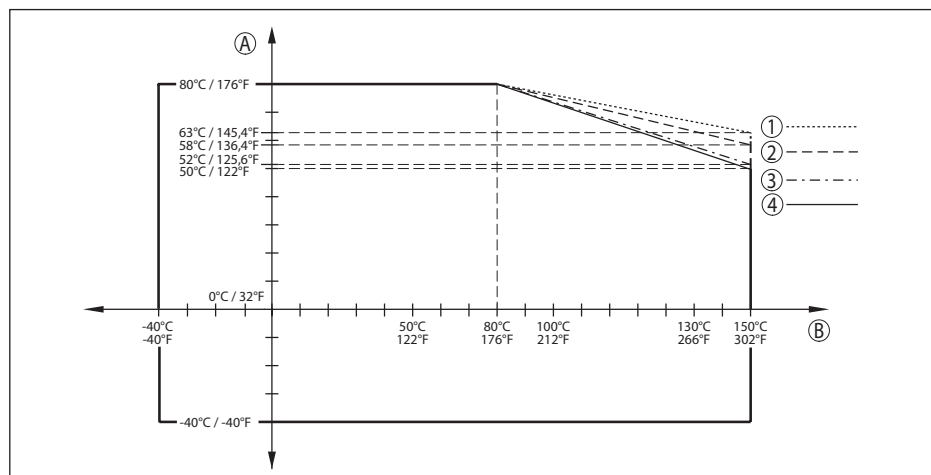
Fig. 68: Derating température ambiante, bride avec antenne lentille jusqu'à +150 °C (+302 °F)
