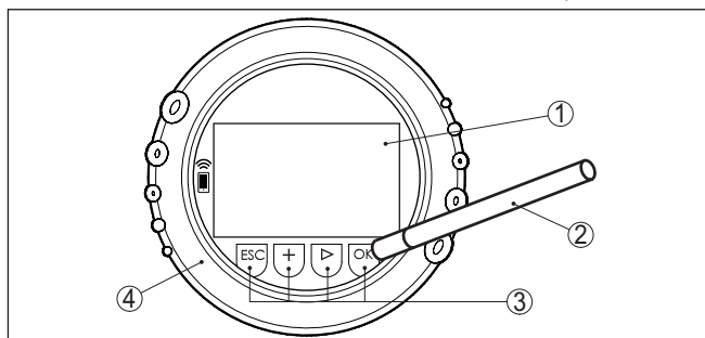
Fig. 51: Éléments de réglage et d'affichage - avec paramétrage par le stylet
