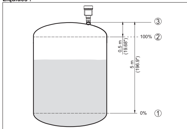
Fig. 52: Exemple de paramétrage du réglage min./max. - Liquides
