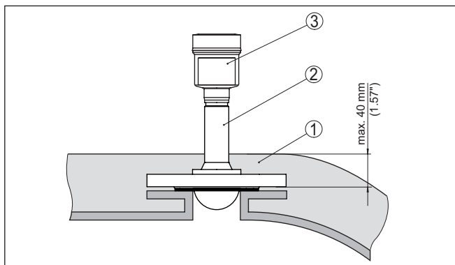
Fig. 28: Montage de l'appareil dans des cuves isolées
