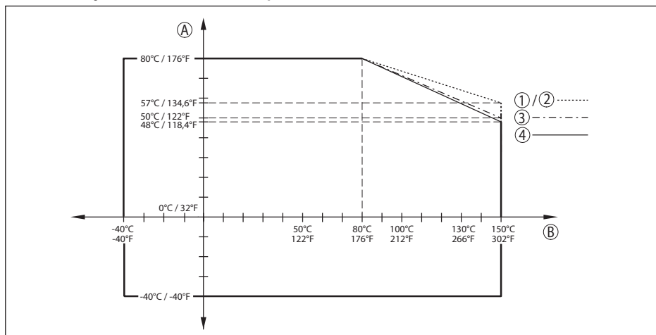
Fig. 64: Derating température ambiante, bride avec système d'antenne encapsulé jusqu'à +150 °C (+302 °F)
