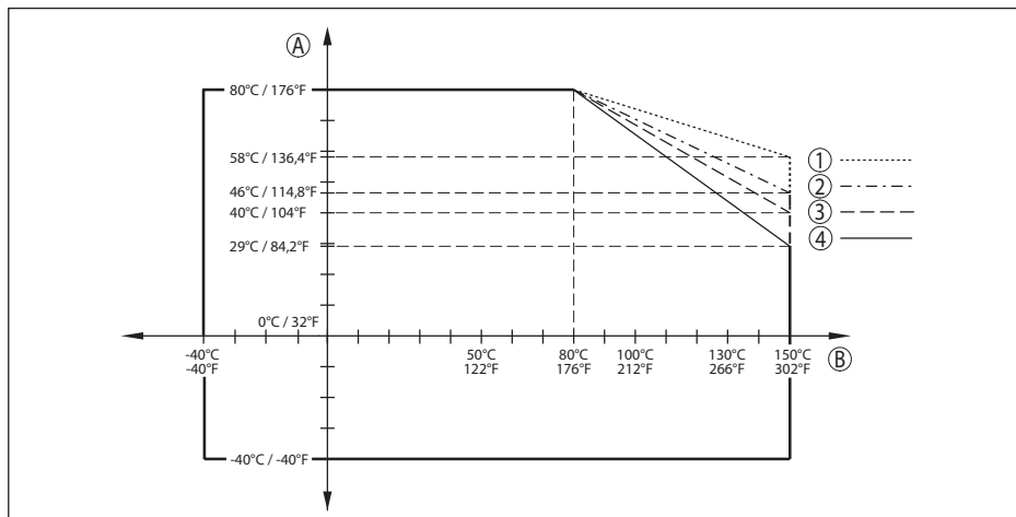
Fig. 72: Derating température ambiante, bride avec antenne cône jusqu'à +150 °C (+302 °F)
