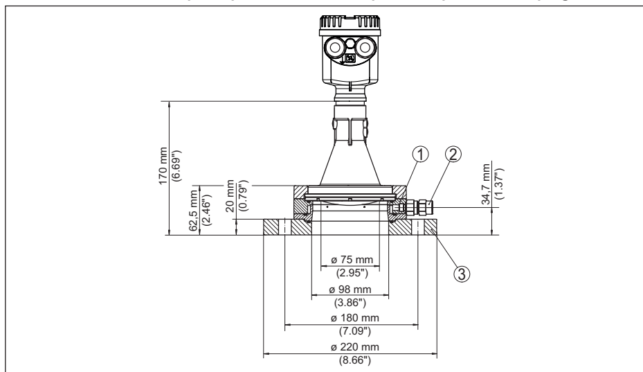
Fig. 81: NCR-86, bride d'adaptation et prise d'air de purge DN 100 PN 6
