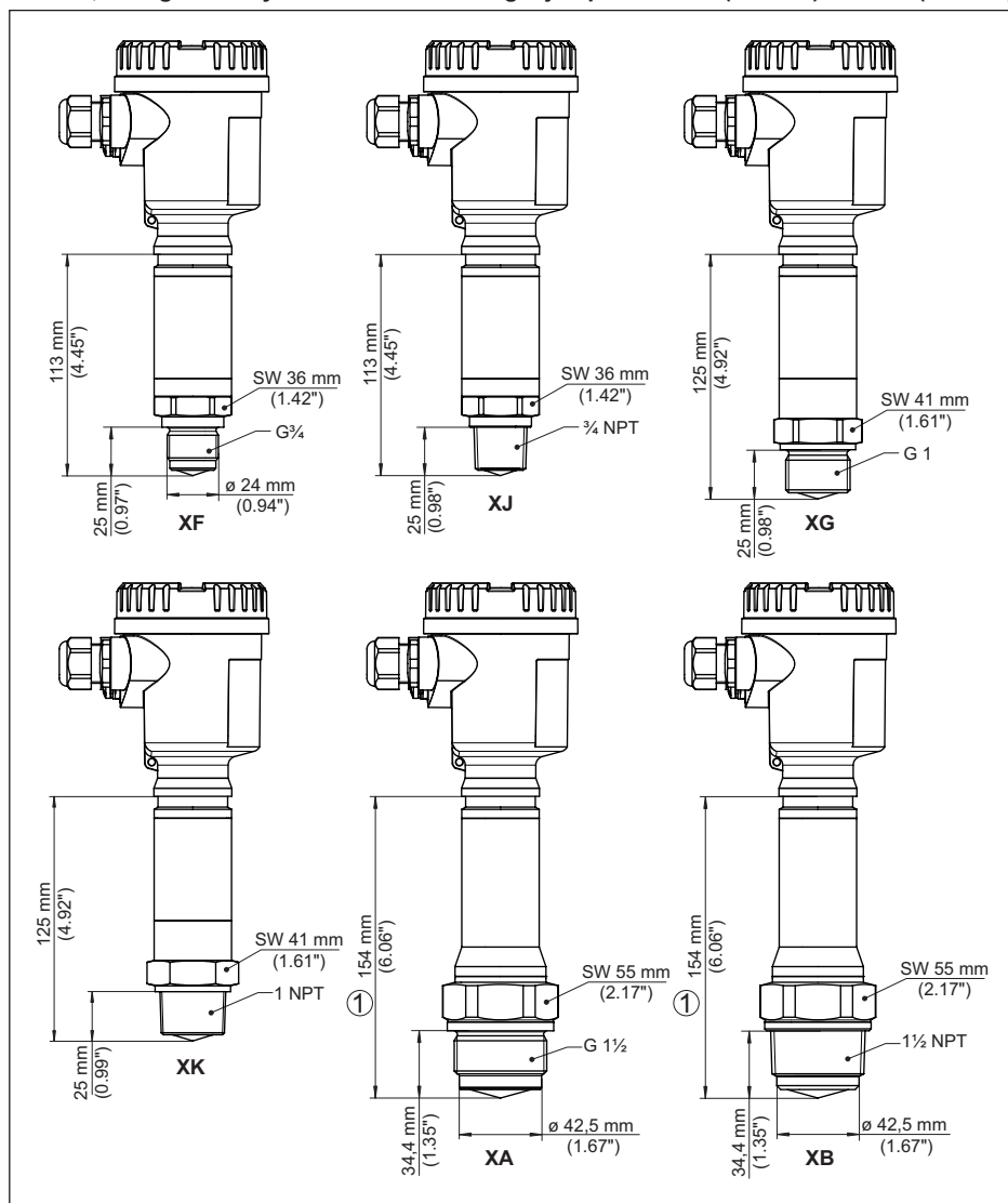
Fig. 85: NCR-86, filetage avec système d'antenne intégré jusqu'à +200 °C (+392 °F)/+250 °C (+482 °F)
