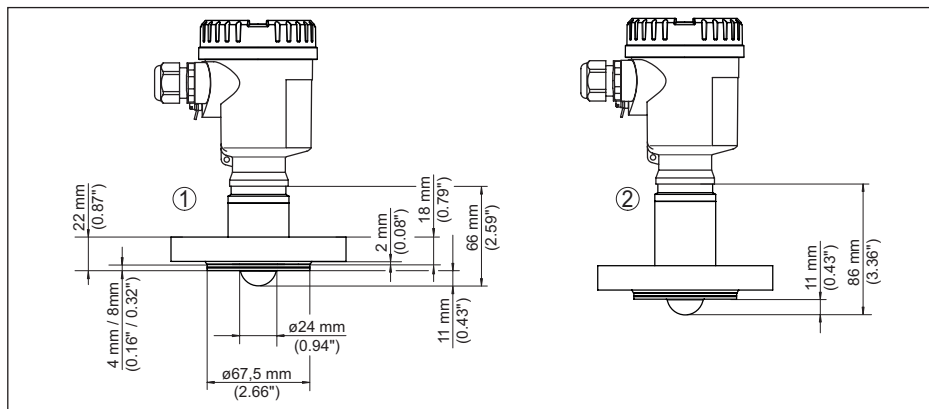
Fig. 89: NCR-86, système d'antenne encapsulé DN 25 PN 40
