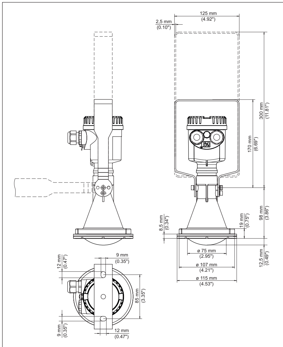
Fig. 82: NCR-86, antenne cône en plastique, support de montage en 170 ou 300 mm de longueur
