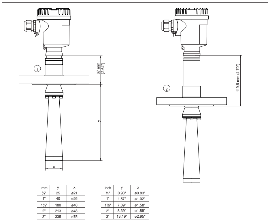
Fig. 86: NCR-86, bride avec antenne cône jusqu'à +150 °C (+302 °F)/+250 °C (+482 °F)
