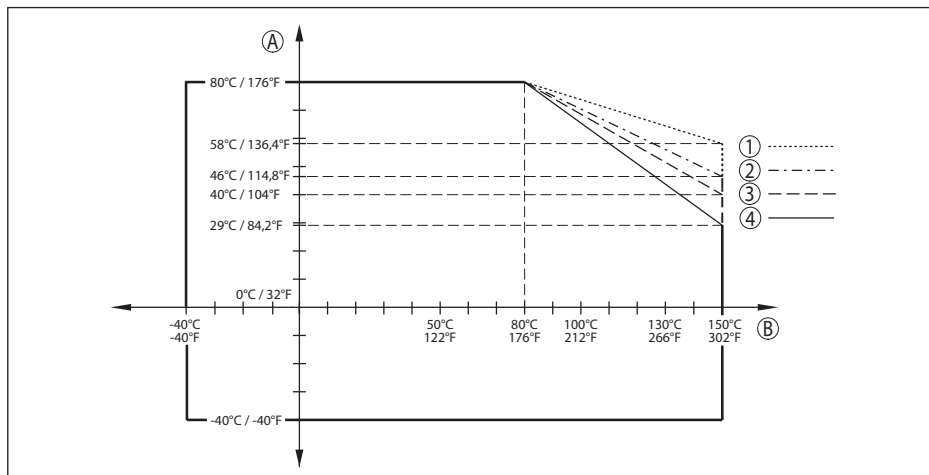
Fig. 61: Derating température ambiante, filetage avec système d'antenne intégré jusqu'à +150 °C (+302 °F)
