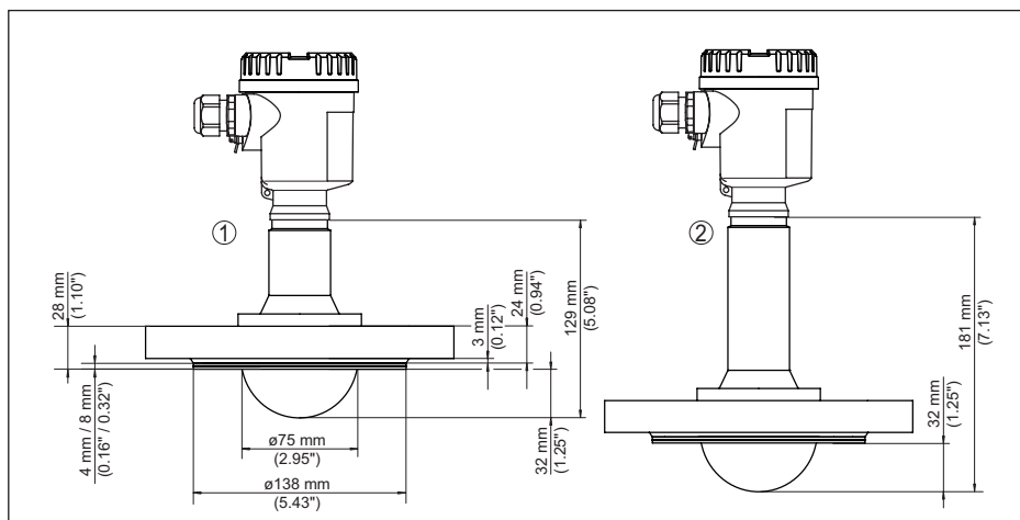
Fig. 90: NCR-86, système d'antennes encapsulé DN 80 PN 40
