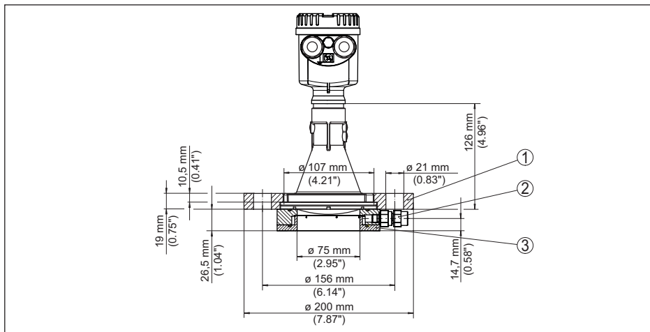
Fig. 79: NCR-86 avec bride tournante et prise d'air de purge pour 3" 150 lbs, DN 80 PN 16
