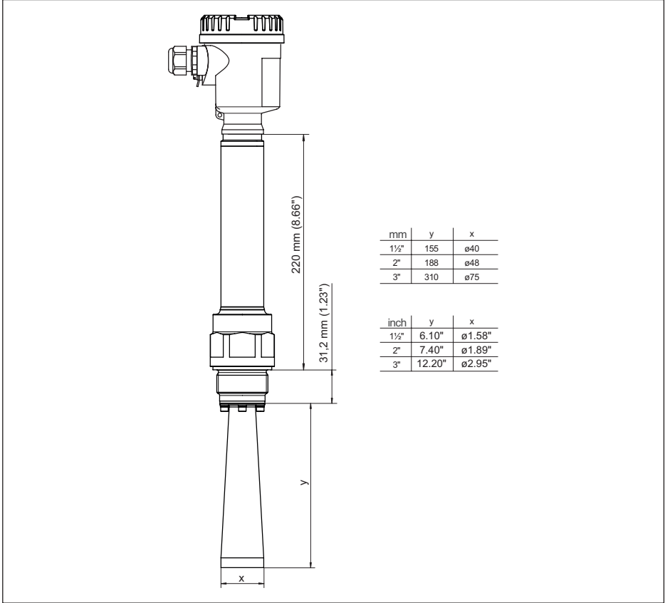
Fig. 87: NCR-86, filetage avec antenne cône version 450 °C
