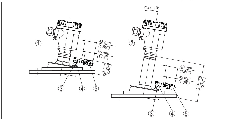
Fig. 97: NCR-86, bride avec antenne lentille, rotule d'orientation et prise d'air de purge
