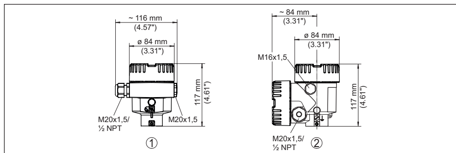
Fig. 76: Variantes de boîtier en protection IP66/IP68 (0,2 bar), (avec un module de réglage et d'affichage intégré, la hauteur du boîtier augmente de 18 mm/0.71 in)
