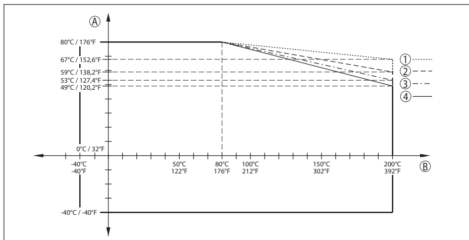
Fig. 62: Derating température ambiante, filetage avec système d'antenne intégré jusqu'à +200 °C (+392 °F)
