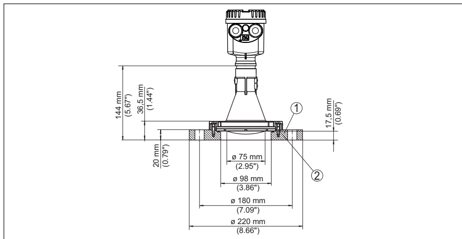
Fig. 80: NCR-86 avec bride d'adaptation DN 100 PN 6
